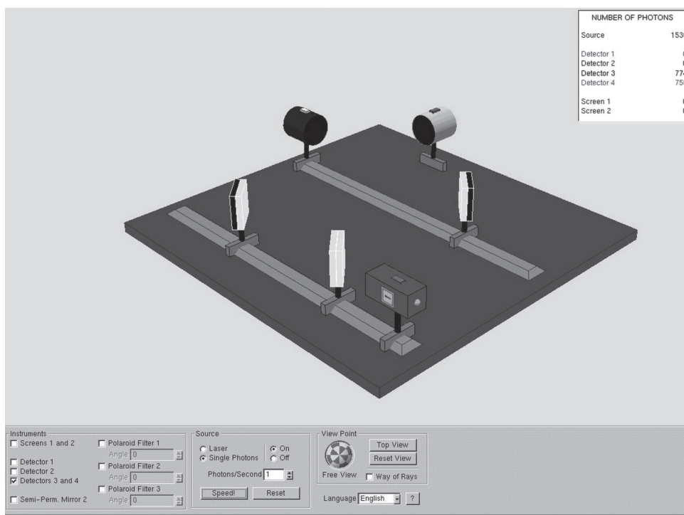
Figura 1. Verificando a indivisibilidade dos fótons.
