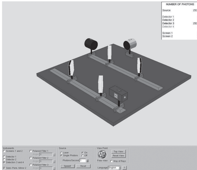
Figura 2. Interferência para fótons únicos.
