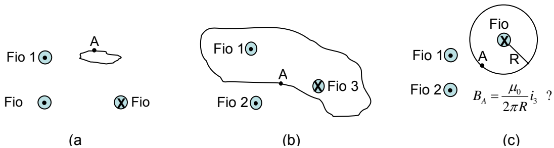
Figura B5.- Seção transversal de três fios retos longos conduzindo corrente e um laço amperiano: (a) não envolvendo os fios; (b) envolvendo os fios 1 e 3; c) envolvendo apenas o fio 3, sendo mostrada a expressão para o campo magnético resultante num ponto "A" a uma distância "R" deste fio.
