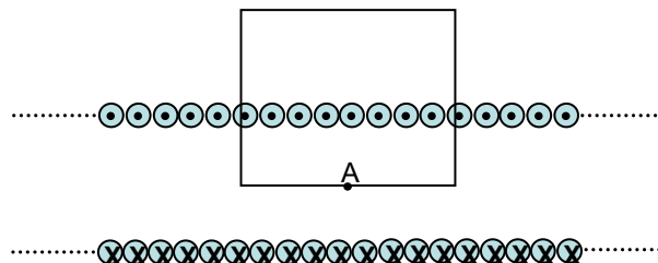
Figura B6.- Vista em corte de um solenóide ideal infinito, com uma região envolvida por uma curva de integração retangular.
