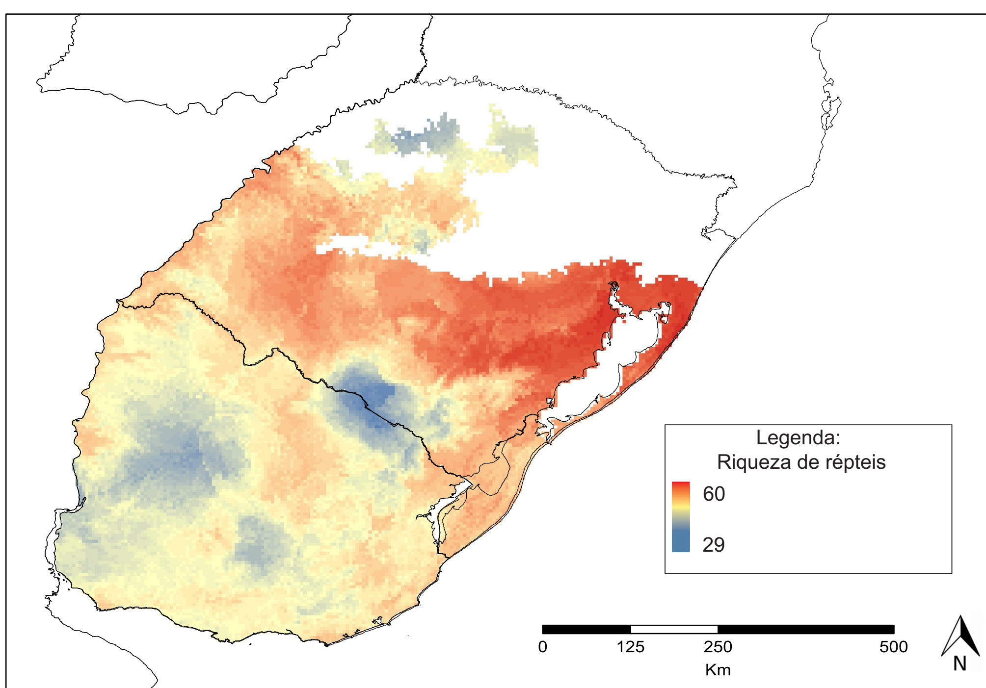
Figura 1: Modelo potencial de riqueza de espécies de répteis para a Savana Uruguaia usando o limiar "minimum presence".
