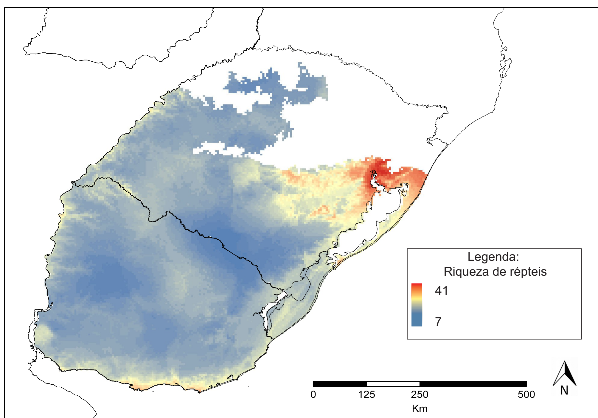
Figura 3: Modelo potencial de riqueza de espécies de répteis para a Savana Uruguaia usando o limiar "Equal training sensitivity and specificity"
