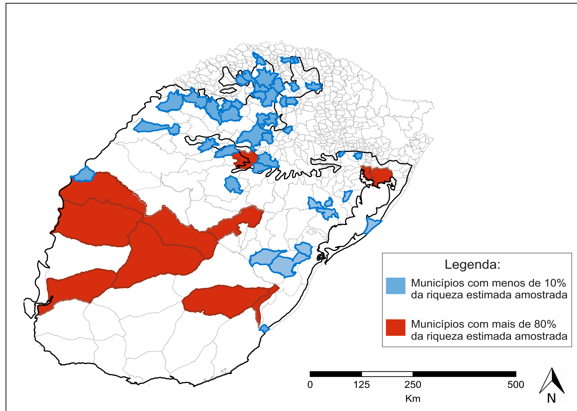
Figura 2: Municípios da Savana Uruguaia que obtiveram menos de 10% da riqueza amostrada em comparação com o modelo, e mais de 80% da riqueza amostrada, para o limiar minimum presence - MNP.
