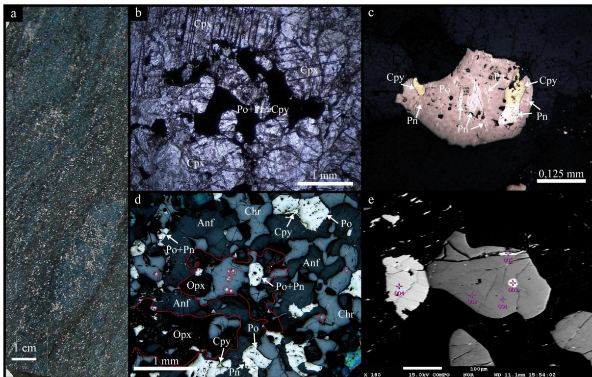
Figura 28: Feições da mineralização sulfetada magmática. (a) Testemunho de sondagem de piroxenito anfibolitizado com forte sulfetação disseminada. (b) Sulfetos nos intersticiais em clinopiroxênio cúmulus-intercúmulus. (c) Típica ocorrência dos sulfetos, intercrescimentos de pirrotita+calcopirita+pentlandita e exsoluções flame de pentlandita em pirrotita. (d) Intercrescimentos de sulfetos, anfibólio, cromoespinélio e ortopiroxênio esquelético. Inclusões de sulfetos no cromoespinélio destacadas pelas elipses. (e) Imagem de elétrons retroespalhados de sulfetos e cromoespinélio onde foram realizadas análises EDS. Cpx=clinopiroxênio, Opx=ortopiroxênio, Po=pirrotita, Pn=pentlandita, Cpy=calcopirita, Anf=anfíbólio. (b) NP, (c, d) luz refletida.
