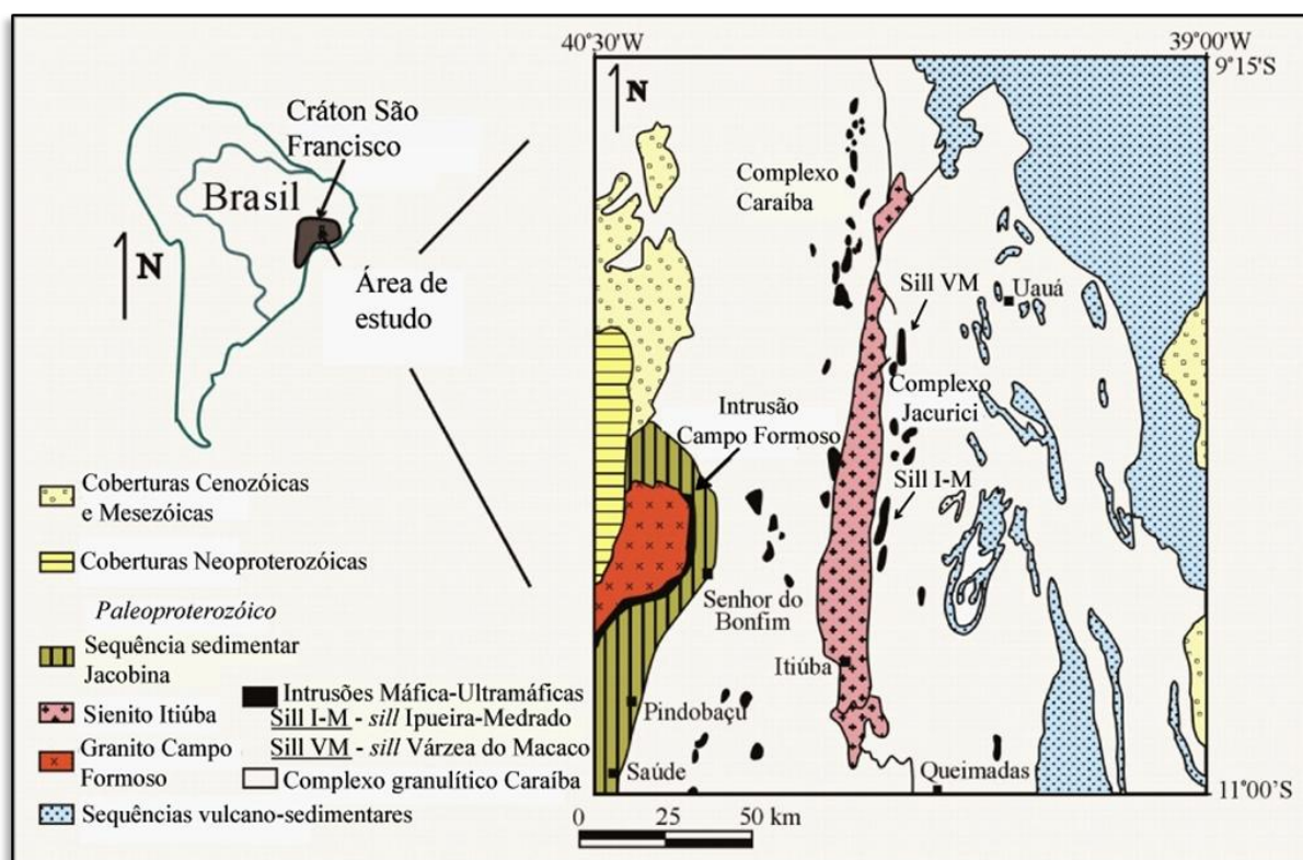
Figura 16: Localização da área de estudo e geologia da região. O Complexo Máfico-ultramáfico Jacurici e o Complexo Caraíba são separados pelo Sienito Itiúba. (modificado de Marques et al. 2005).
