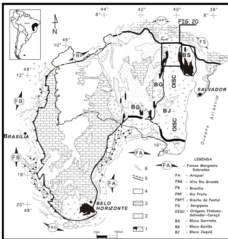
Figura 19: Mapa do Cráton do São Francisco. 1. Embasamento Arqueano/Paleoproterozóico com seqüências greenstone belts e o Grupo Jacobina (em preto); 2. Coberturas Mesoproterozóicas do Supergrupo Espinhaço 3. Coberturas Neoproterozóicas do Supergrupo São Francisco; 4. Coberturas Fanerozóicas; 5. Limites do Cráton (Ussami 1993); 6. Cinturões de dobramentos Brasileiros. A região estudada está na área destacada (Modificado de Barbosa et al. , 2003b).
