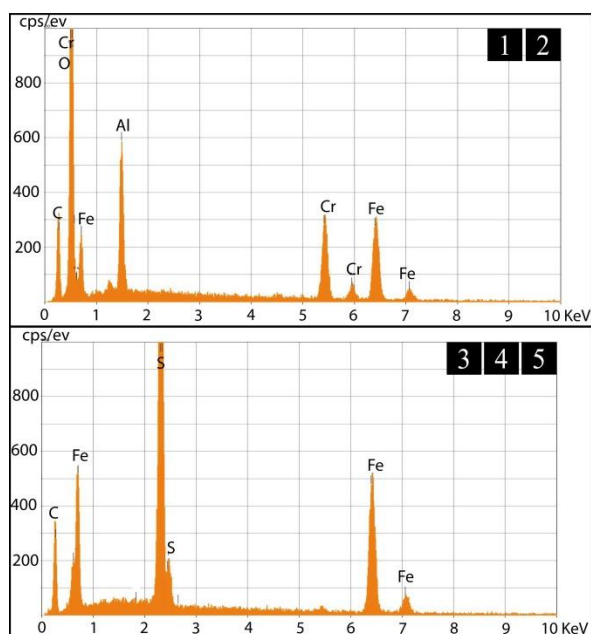
Figura 29: Análises EDS da Fig. 28e. (1, 2) Composição do cristal de cromita. (3, 4, 5) Composição das inclusões de pirrotita. Análises estão agrupadas porque os espectros se sobrepõem.
