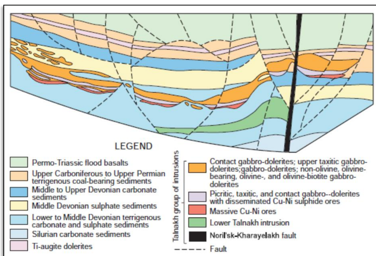
Figura 4: Seção geológica oeste-leste de Noril'sk (extraído de Eckstrand & Hulbert, 2007).
