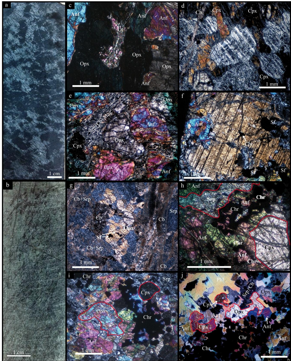
Figura 24: Feições do Iherzolito. (a) Testemunho com porções esbranquiçadas onde ocorrem minerais preservados da serpentinização. (b) Lherzolito anfibolitizado em zona metassomática/hidrotermal. Faixas de cristais escuros são lentes de Cr-espínélio. (c) Olivina inclusa em ortopiroxênio (ext. levemente ondulante) intercrescido com anfibólio magmático que exhibe exsoluções lamelares (indicadas pelas setas). (d) Textura cumulática somente com cristais intercúmulus preservados, interceptados por veio de carbonato. (e) Anfibólio magmático intercrescido com piroxênios. (f) Ortopiroxênio de aspecto esqueletal com inclusão de cromoespinélio e pirrotita±pentlandita associado a anfibólio. (g) Lherzolito afetado por carbonatação. Relictos de ortopiroxênio incluem pirrotita±pentlandita magmáticas. (h) Clinopiroxênio com anfibolitização secundária nas bordas. Cromoespinélio de textura em rede remete à textura ígnea. (i) Clinopiroxênio associado a anfibólio em substituições parciais irregulares e cromoespinélio de textura em rede. (j) Relictos de piroxênios magmáticos esqueletais e camada diminuta de cromitito em zona intensamente metassomatizada com flogopita+anfibólio±carbonato. Ol=olivina, Opx=ortopiroxênio, Cpx=clinopiroxênio, Anf=anfibólio, Chr=cromita/cromoespinélio, Sf=sulfetos, Srp=serpentina, Cb=carbonato, Phl=flogopita. Fotomicrografias em NX.
