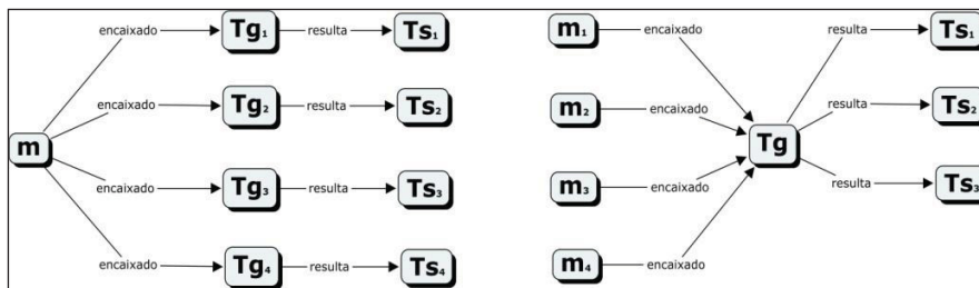
Fig. 2 – À esquerda, um modelo conceitual ( m ) acolhido por quatro teorias gerais distintas ( Tg_1, Tg_2, Tg_3, Tg_4 ) resulta em quatro teorias específicas ou modelos teóricos ( Ts_1, Ts_2, Ts_3, Ts_4 ) distintos; à direita, quatro modelos conceituais ( m_1, m_2, m_3, m_4 ) acolhidos pela mesma teoria geral ( Tg ) resultam em três teorias específicas ( Ts_1, Ts_2, Ts_3 ). O número de teorias gerais (à esquerda) e de modelos conceituais (à direita) é meramente ilustrativo. Além disso, nem todo modelo conceitual dá origem a um modelo teórico.
