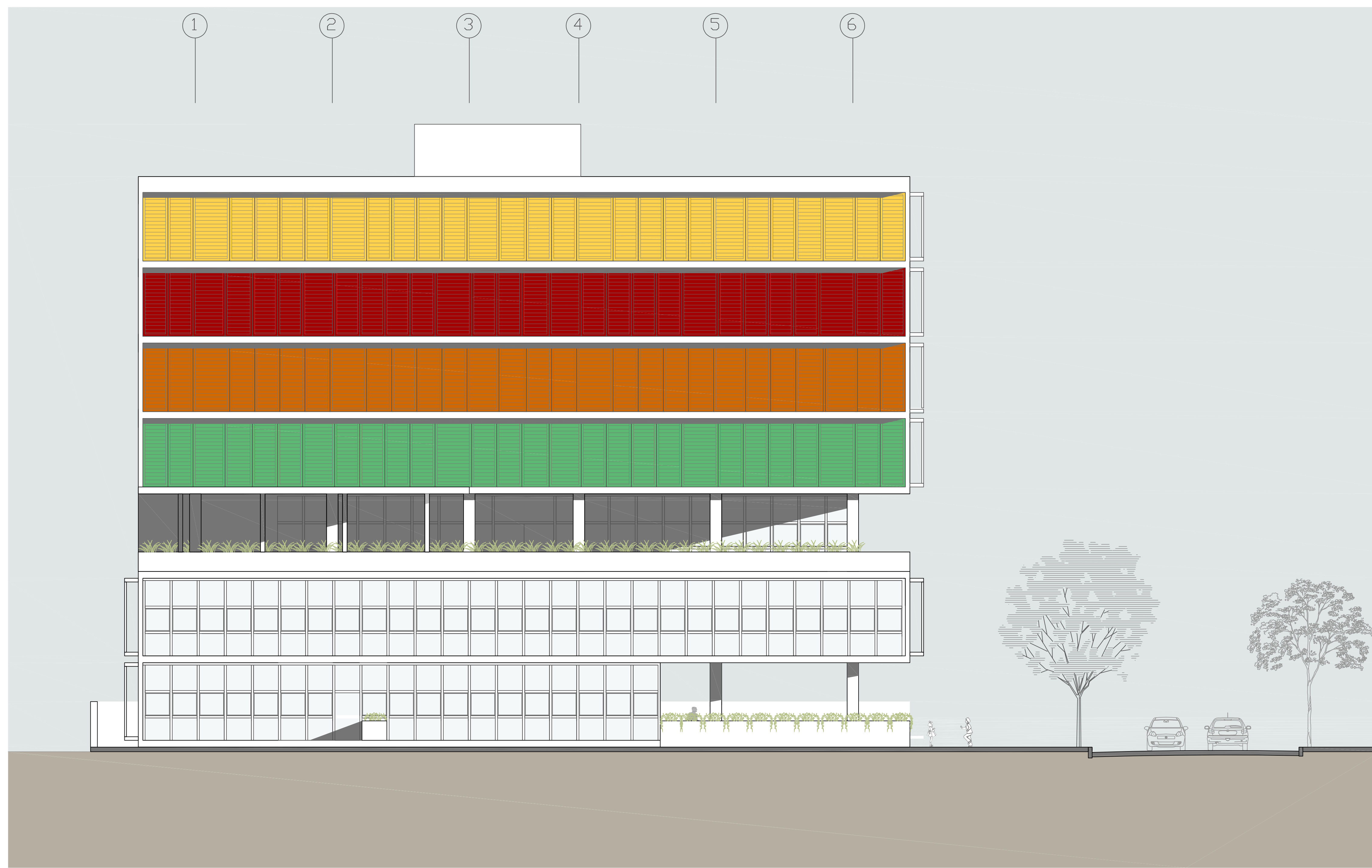
FACHADA NORTE 1/100
