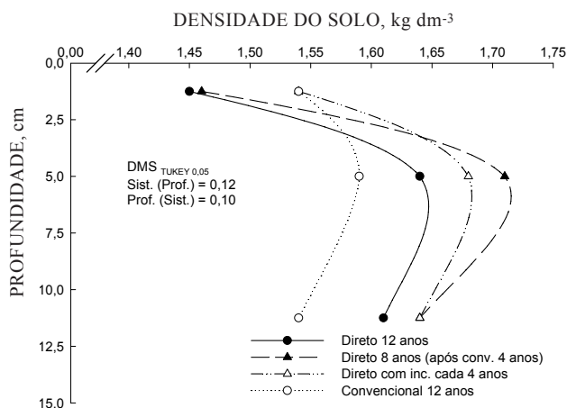
Figura 1. Densidade do solo em diferentes sistemas de manejo e profundidades.
