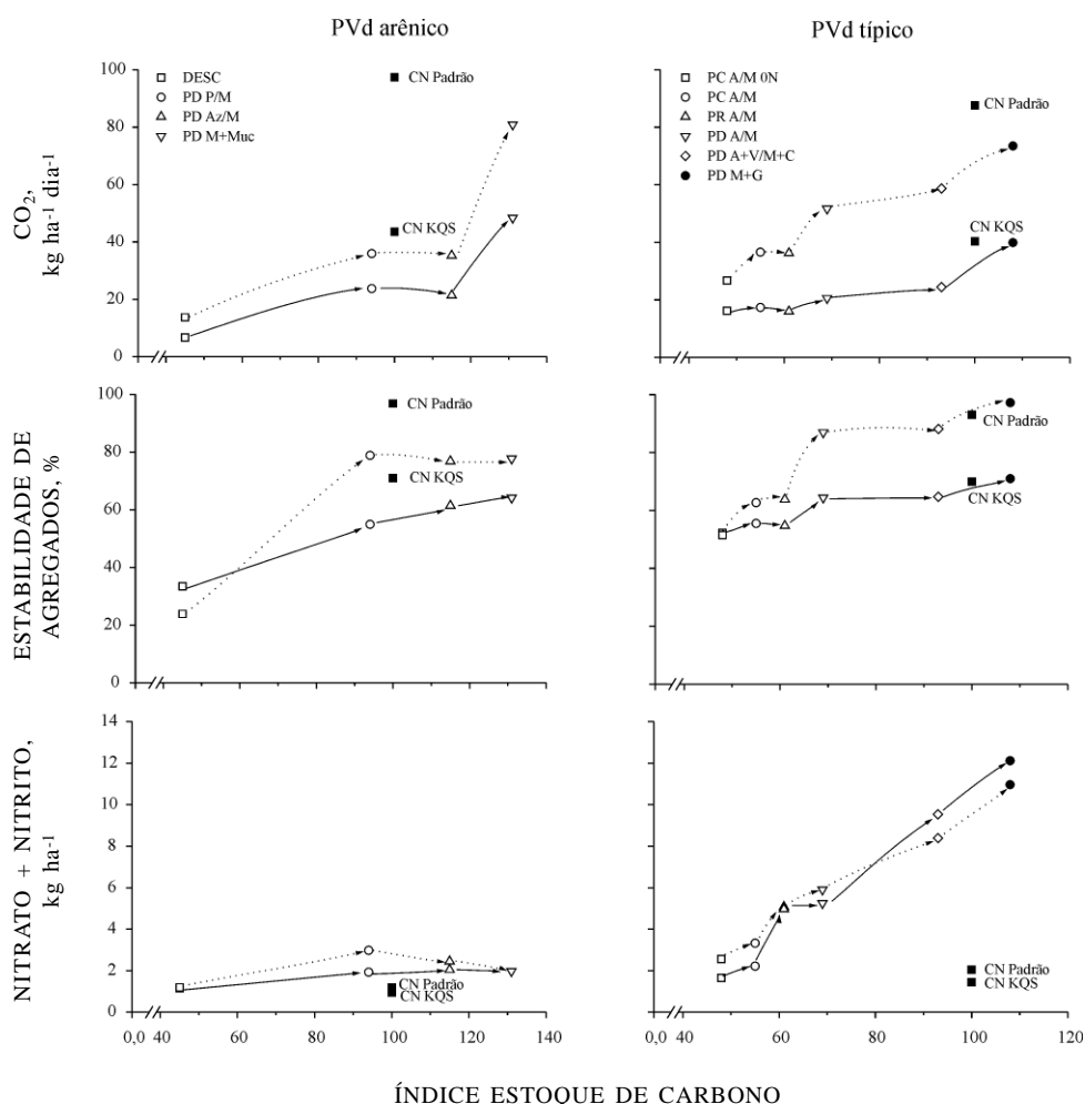
Figura 2. Relação entre o Índice de Estoque de Carbono (IEC) e os indicadores respiração do solo (CO 2 ), estabilidade de agregados em água e nitrato+nitrito, avaliados pelos métodos padrão (linha pontilhada) e do kit de qualidade do solo (linha cheia). DESC. = solo descoberto; CN = campo natural; PC = preparo convencional; PR = preparo reduzido; PD = plantio direto; Az = azevém; P = pousio; Muc = mucuna; A = aveia; M = milho; V = ervilhaca; C = caupi; G = guandu e 0N = sem adubação nitrogenada. PVd arênico = Argissolo Vermelho distrófico arênico; PVd típico = Argissolo Vermelho distrófico típico.
