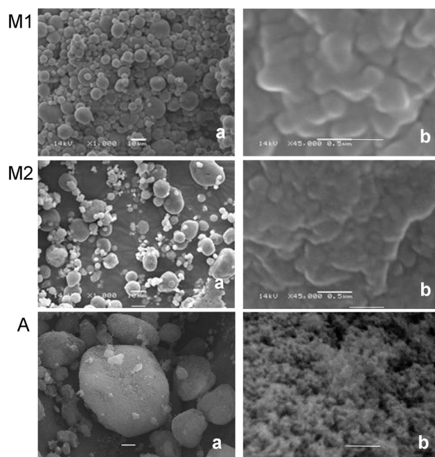
Figura 3. Fotomicrografias das formulações de micropartículas nanorevestidas M1 (PCL) e M2 (ERS); e do Aerosil ® 200 (A) [(a) largura da barra 10 µm, (b) largura da barra 0,5 µm]
