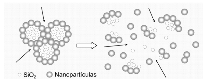
Figura 5. Esquema do mecanismo de desaglomeração a partir das micropartículas nanorevestidas, as setas indicam a penetração do solvente
