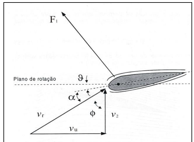
Figura 3: Relações entre ângulos, força e velocidades em um perfil aerodinâmico. Fonte: [8].
