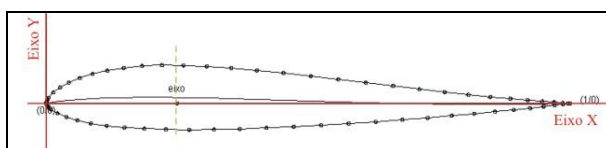
Figura 2: Forma do perfil aerodinâmico MH110
