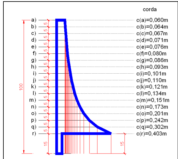
Figura 4: Dimensões da corda c da pá para as seções definidas
