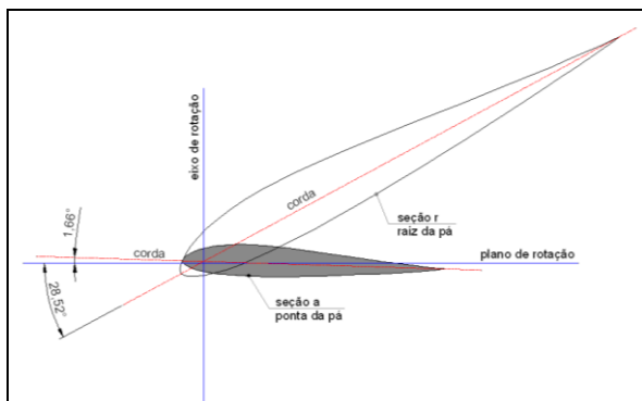
Figura 6: Primeiro e último ângulos de passo da pá
