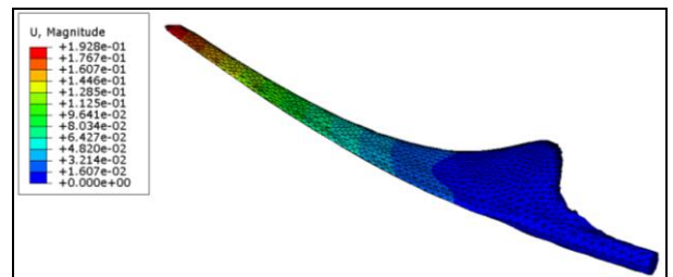
Figura 10: Deslocamento na pá em m
