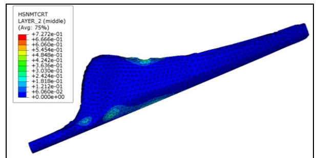
Figura 12: Resultados do critério de falha de Hashin para tração na matriz
