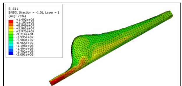
Figura 11: Tensões \sigma_{11} (direção do eixo longitudinal da pá)
