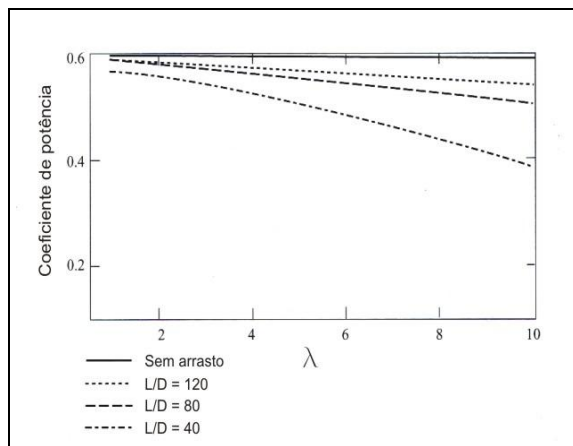
Figura 1: Sustentação (L) e arrasto (D) em função do coeficiente de potência e velocidade específica. Fonte: [3]
