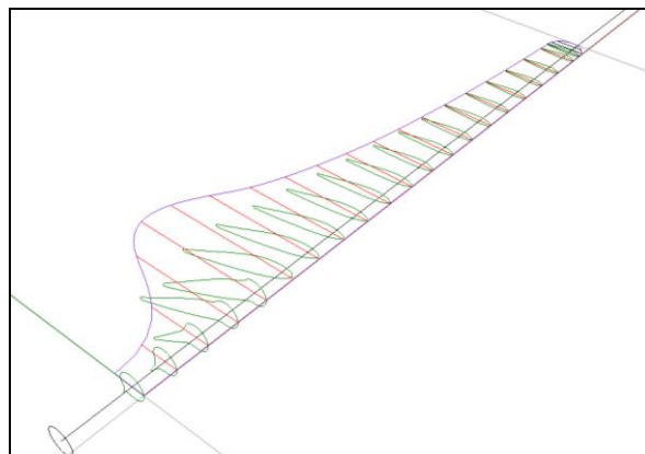
Figura 8: Modelo com perfil aerodinâmico e twist
