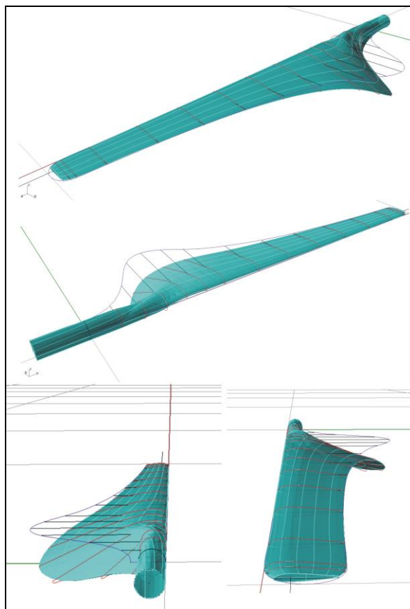
Figura 9: Pá com superfície
