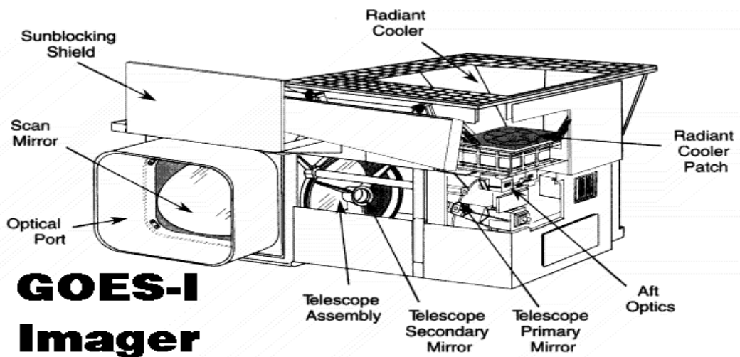
Figura II.7 – Imageador GOES (6)
