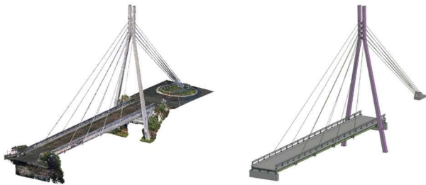
Figura 3 - Construção do modelo 3D de Mohammadi et al. (2023) a partir de nuvem de pontos de Laser Scanning .
