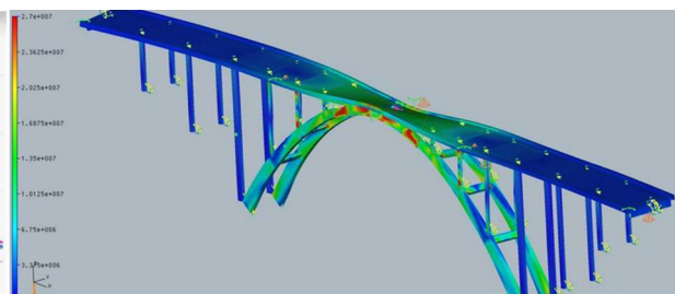
Figura 2 - Modelo do comportamento da ponte após o incidente (Hagen e Andersen, 2024)
