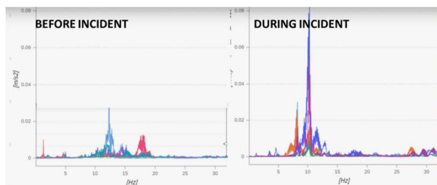
Figura 1 - Sinal dos sensores antes e durante o incidente (Hagen e Andersen, 2024).
