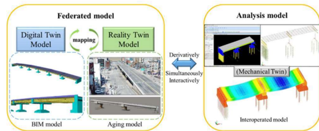
Figura 4 - Conceito de um DT voltado para manutenção de pontes, conforme Shim et al. (2019)
