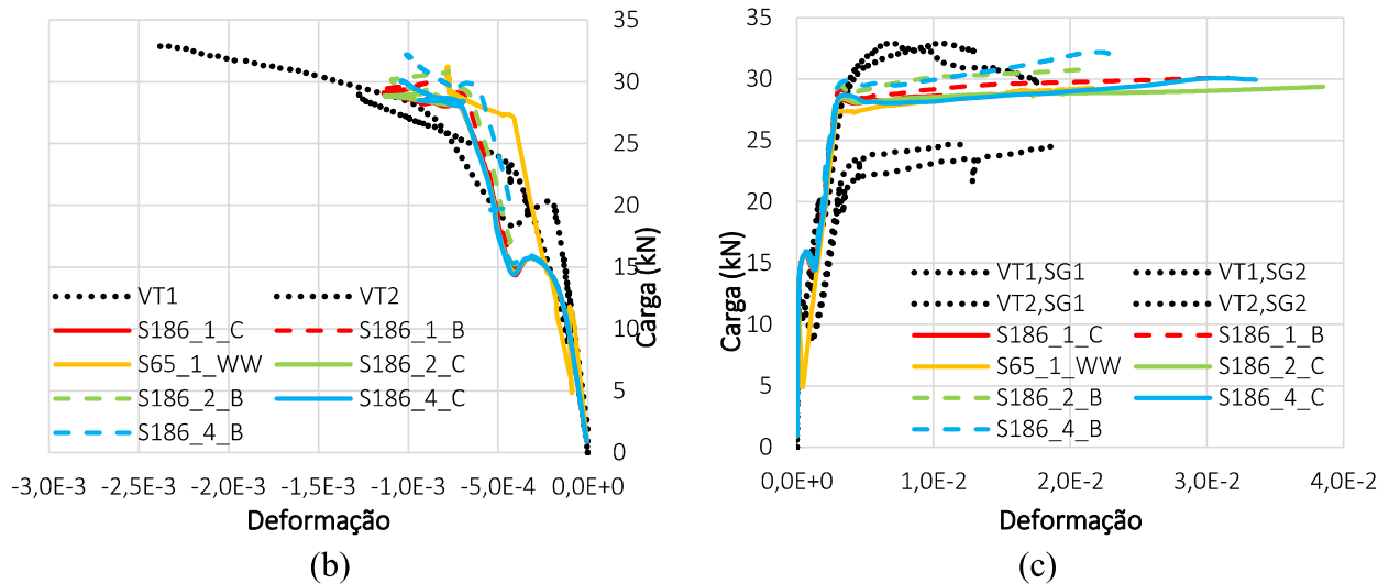
Figura 8 – Posição de coleta de dados; Gráfico carga x deformação: (b) concreto e (c) aço
