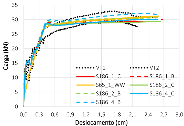
Figura 7 – Gráfico carga x deslocamento VT
