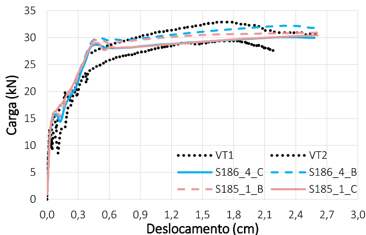
Figura 9 – Gráfico carga x deslocamento SOLID 185
