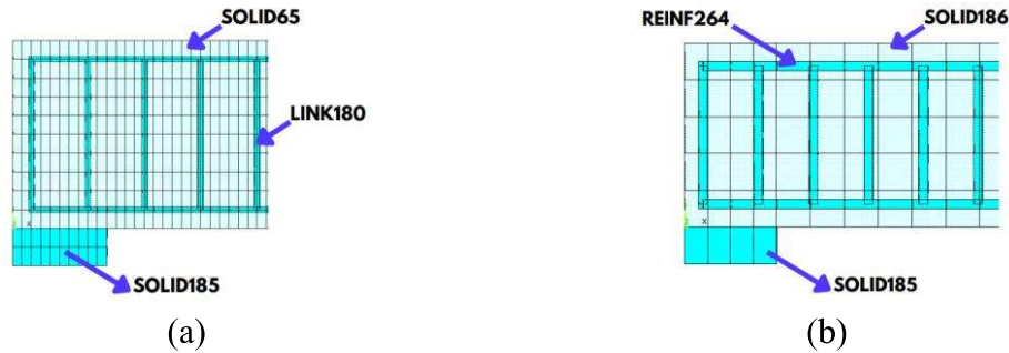
Figura 2 – Armadura (a) Discreta e (b) Incorporada
