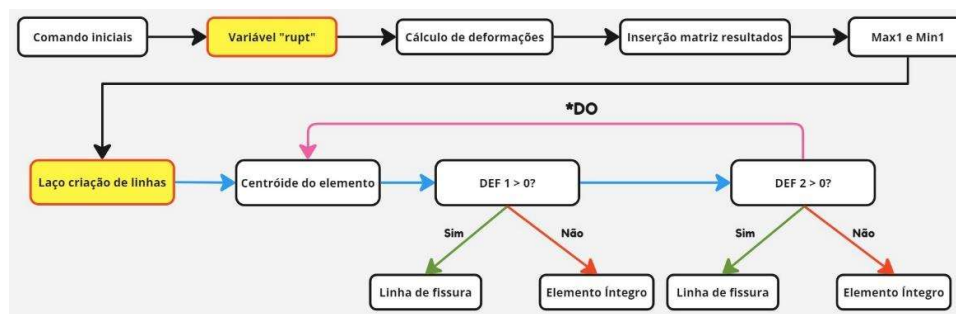
Figura 6 – Fluxograma do script
