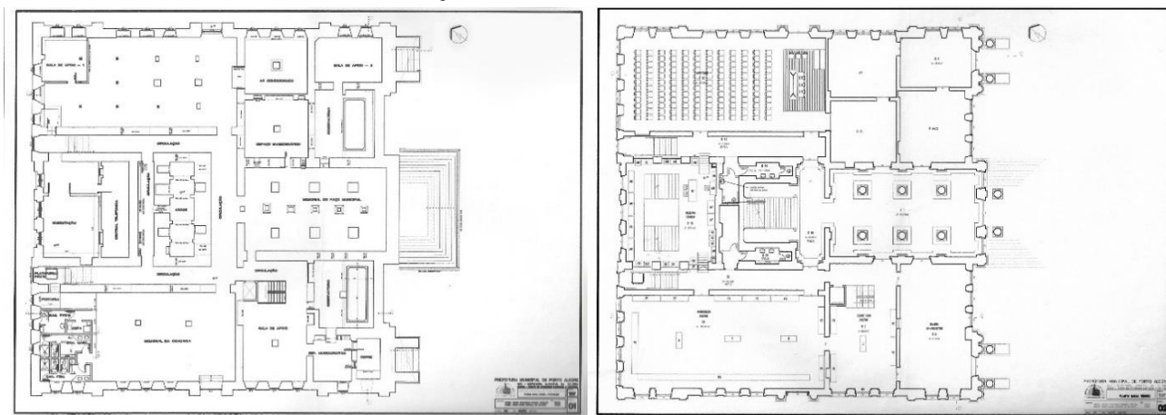
Figura 6 - Planta baixa do subsolo e térreo.
