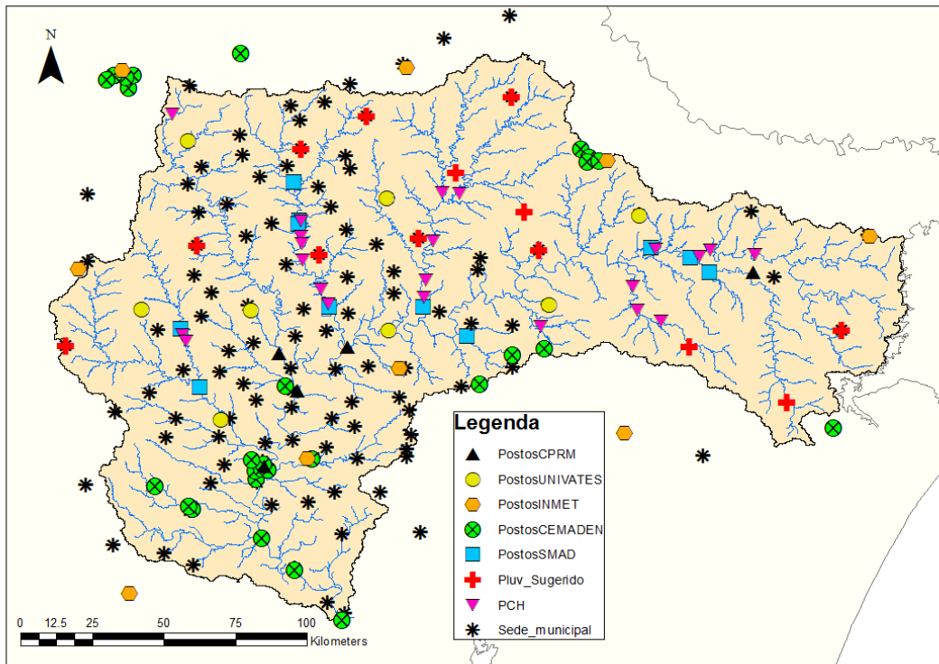
Figura 20 - Mapa de monitoramento pluviométrico hipotético na bacia do rio Taquari-Antas considerando os postos existentes atualmente (CEMADEN, UNIVATES, CPRM, INMET, SMAD-RS), postos pluviométricos adicionais sugeridos (cruz vermelha), postos adicionais em aproveitamentos hidrelétricos e postos adicionais em cada sede de município da bacia.
