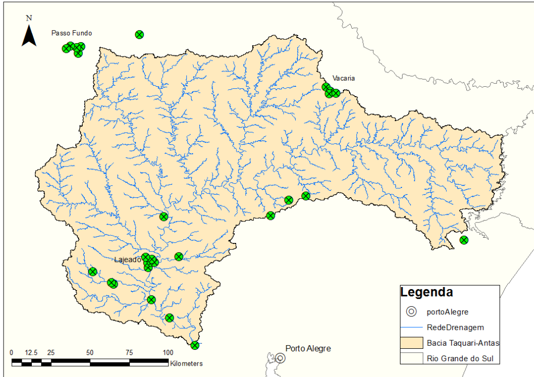
Figura 8 - Localização dos postos pluviométricos telemétricos do CEMADEN instalados na região da bacia do Taquari-Antas no contexto do projeto “Pluviômetros Automáticos” e em operação em setembro de 2015.
