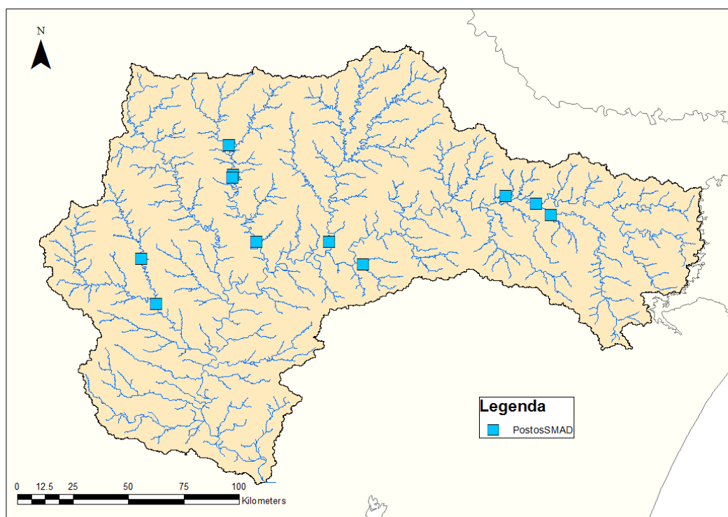
Figura 14 - Mapa de localização dos pontos de monitoramento fluviométrico disponibilizados através do SMAD-RS.
