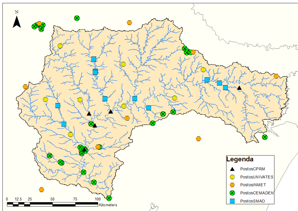
Figura 16 - Rede pluviométrica com telemetria operando atualmente (2015) na bacia do rio Taquari-Antas, incluindo postos do INMET, CPRM, UNIVATES, SMAD-RS e CEMADEN.
