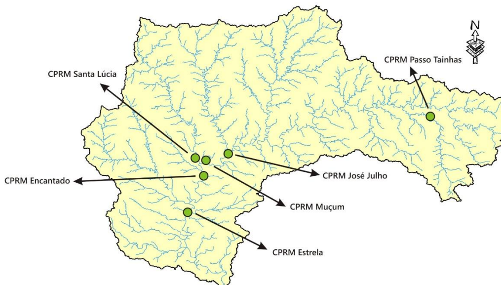
Figura 6 - Localização dos postos pluviométricos telemétricos do sistema SACE da CPRM na bacia do rio Taquari-Antas (não estão ilustrados os postos de Taquari e Mariante, que começaram a operar mais recentemente).
