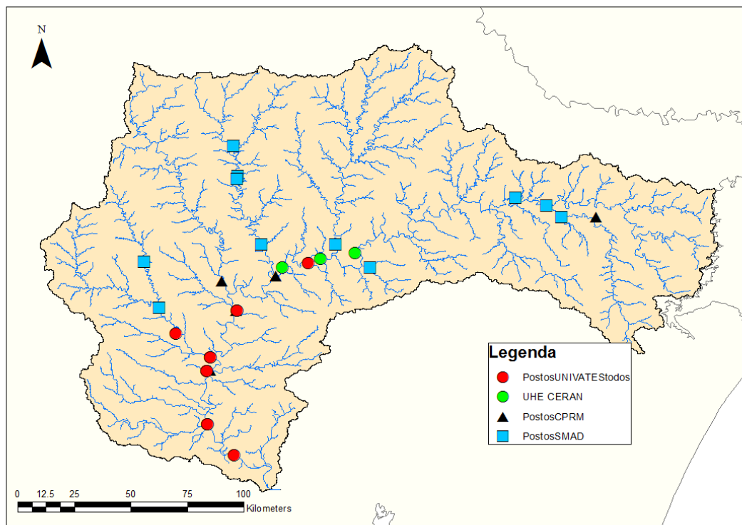
Figura 17 - Mapa de localização dos postos fluviométricos telemétricos atualmente instalados na bacia do rio Taquari-Antas.
