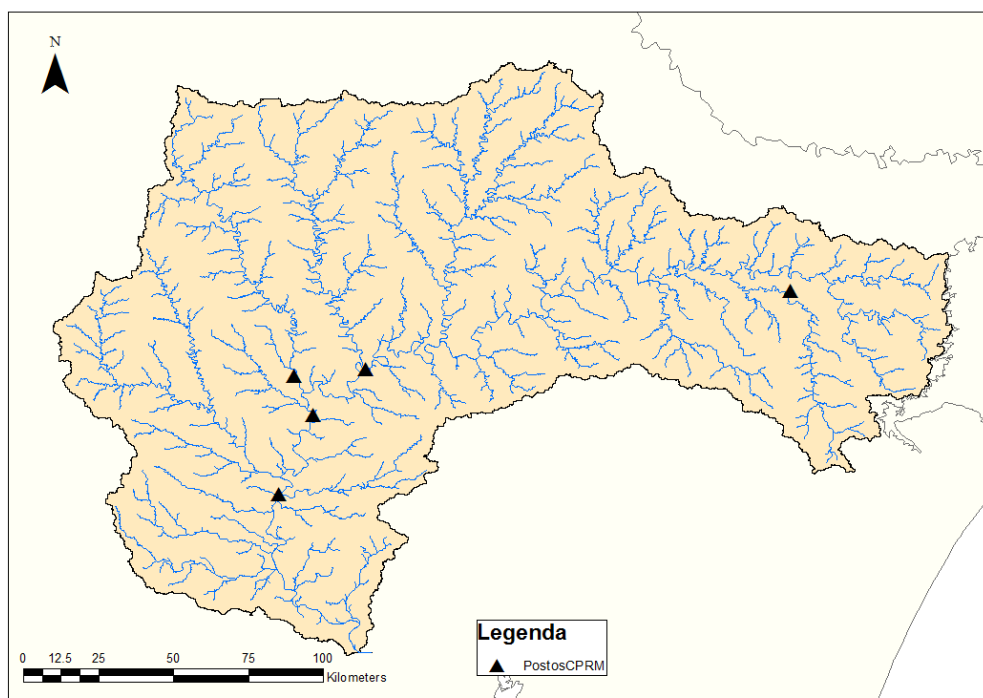
Figura 11 - Mapa de localização das estações fluviométricas da CPRM com telemetria na bacia do rio Taquari-Antas (os postos de Taquari e Mariante não aparecem no mapa porque foram instalados mais recentemente).
