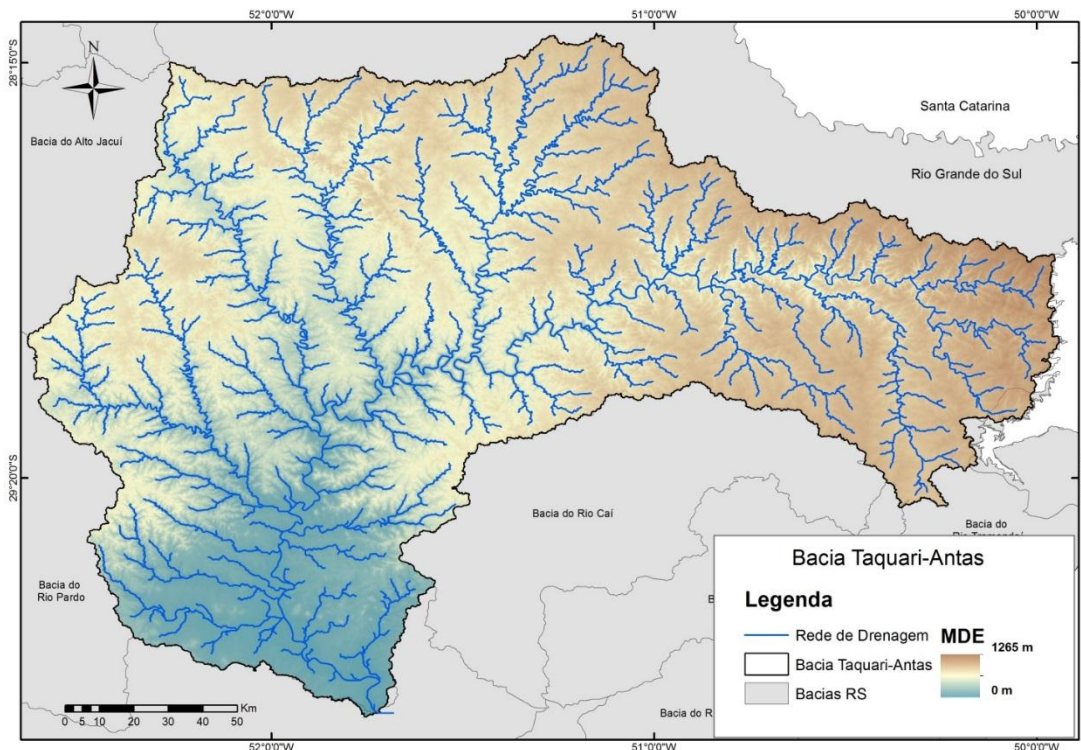
Figura 1 - Relevo da bacia do rio Taquari-Antas (obtido do SRTM com resolução de 90 metros).
