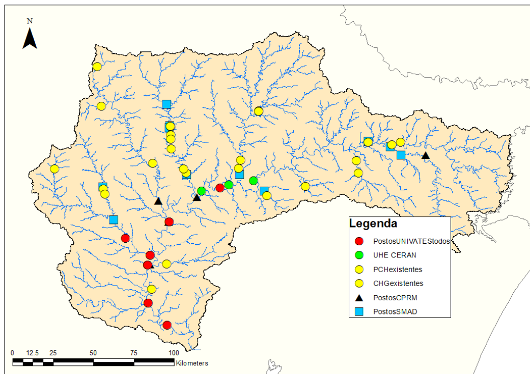
Figura 21 - Postos do monitoramento fluviométrico com telemetria considerando o monitoramento atual e a proposta de instalação e operação de monitoramento em todos os aproveitamentos hidrelétricos atualmente existentes na bacia.
