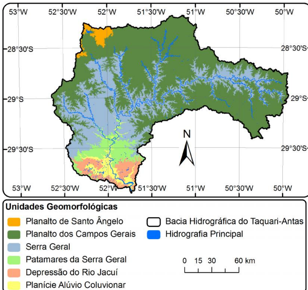
Figura 2 - Unidades Geomorfológicas da bacia hidrográfica do rio Taquari-Antas.
