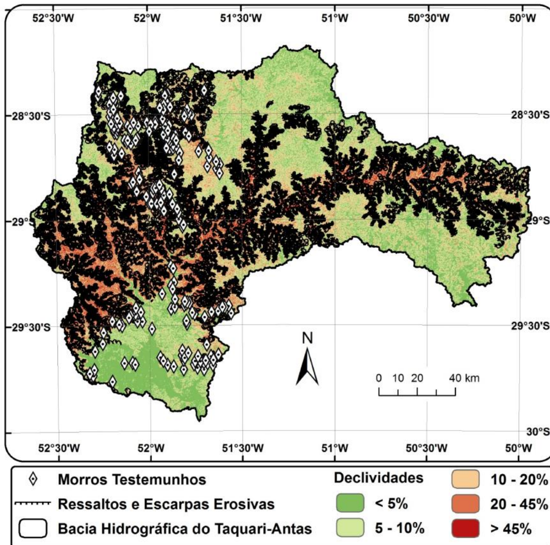
Figura 4 - Ilustração de feições lineares do relevo sobrepostas à base de declividades.
