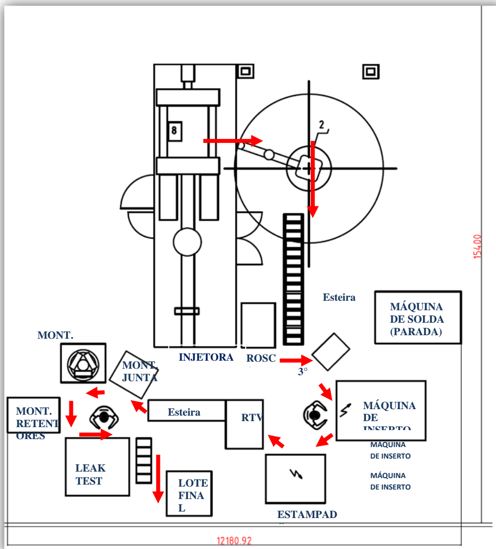
Figura 2 – Layout da célula de manufatura em estudo.
