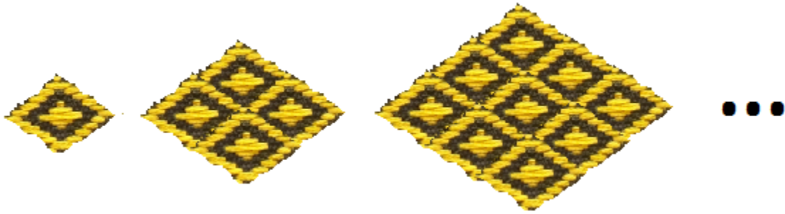
Figura 3– Sequência de números quadrados
