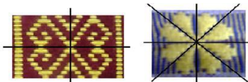
Figura 10 – Os motivos e a reflexão.
