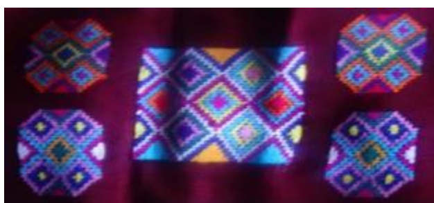
Figura 13 – Os motivos e a dilatação.
