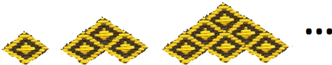
Figura 4 – Outros números triangulares.
