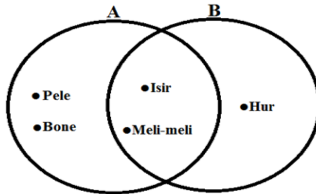
Figura 7 – Tais e a teoria dos conjuntos.
