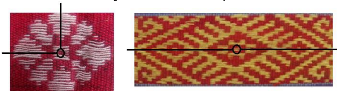
Figura 9 – Os motivos e a rotação.
