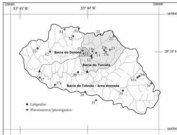
Figura 2 - Localização dos pluviógrafos e pluviômetros utilizados para o cálculo da chuva média, e dos linígrafos de registro de vazão. Observa-se que o linígrafo do Taboão não faz o registro da área total da bacia.
