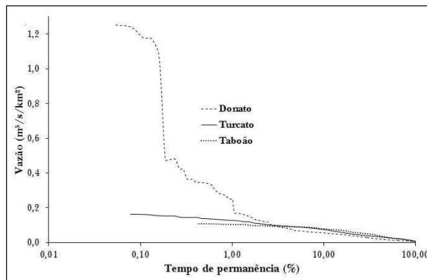
Figura 11 - Curva de permanência de vazões específicas Q 7dias das bacias de estudo.
