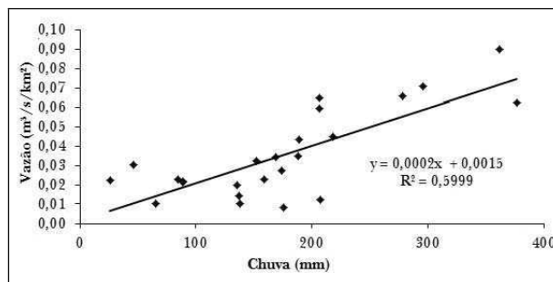
Figura 16 - Relação dos totais de chuva e vazões específicas mensais para a bacia do Taboão.
