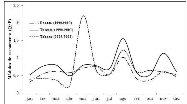
Figura 20 - Módulos de escoamento das bacias do Donato, Turcato e Taboão, pela média dos módulos mensais em cada período.
