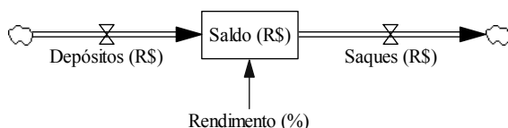
Figura 3 - Exemplo ilustrando uma estrutura bastante usada nos modelos de simulação dinâmica.
