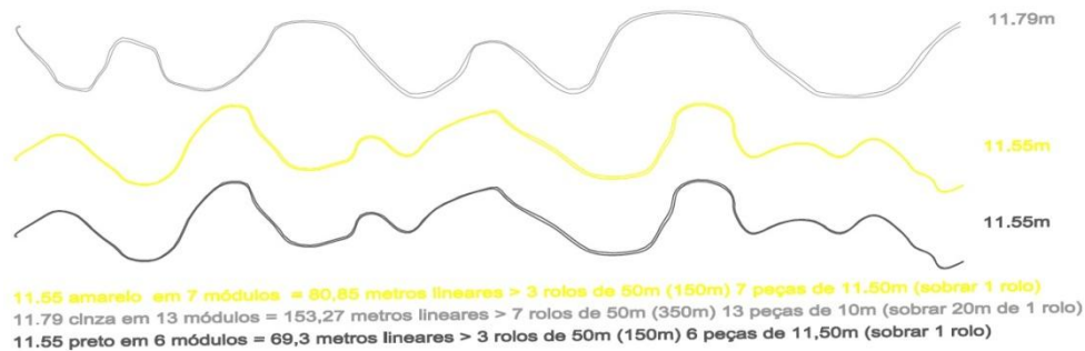
Figura 20: Esquema de cálculo de eletrodutos, em software AutoCad 2007, divididos por cores e multiplicado pelo número de faixas que cada rolo usaria. Fonte: Stefanello Studio .
