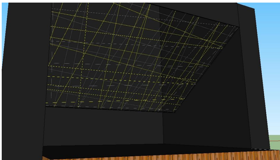
Figura 13: Segunda Proposta, simulação virtual em maquete eletrônica, em software SketchUp 2015 Pro, mostrando a inclinação em ângulo de 35^\circ em relação aos 9 metros de altura da boca de cena. Fonte: Stefanello Studio.
