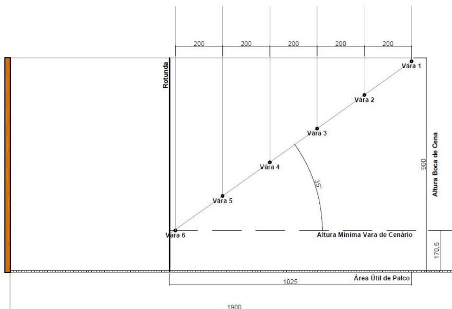
Figura 14: Primeiro Corte, em software AutoCad 2007, mostrando as alturas de cada vara cênica, a inclinação de 35^\circ na estrutura, altura mínima alcançada para manter a angulação, bem como a profundidade de palco utilizada. Fonte: Stefanello Studio.
