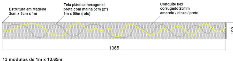
Figura 16: Detalhamento, em software AutoCad 2007, da distribuição de eletrodutos na tela plástica hexagonal. Fonte: Stefanello Studio.
