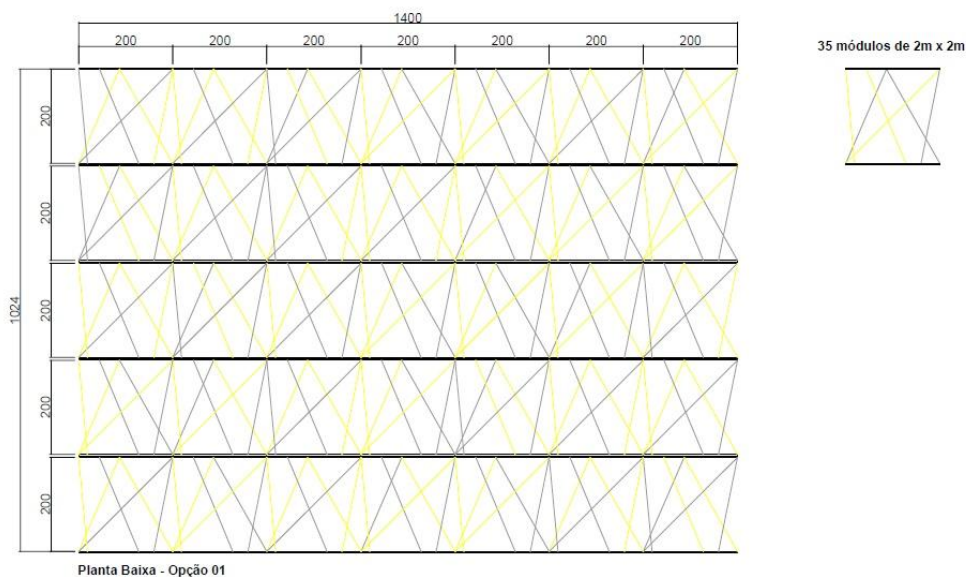
Figura 10: Primeira proposta de planta baixa desenhada em software AutoCad 2007, com 35 módulos de 2m x 2m, formando o preenchimento do palco de 10,24 metros de profundidade e 14 metros de largura. Fonte: Stefanello Studio.
