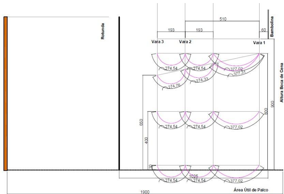
Figura 19: Último corte esquemático, produzido em software AutoCad 2007, mostrando o uso final das 4 varas cônicas, bem como o tamanho de cada secção e o abaulamento estrutural entre varas. Fonte: Stefanello Studio.
