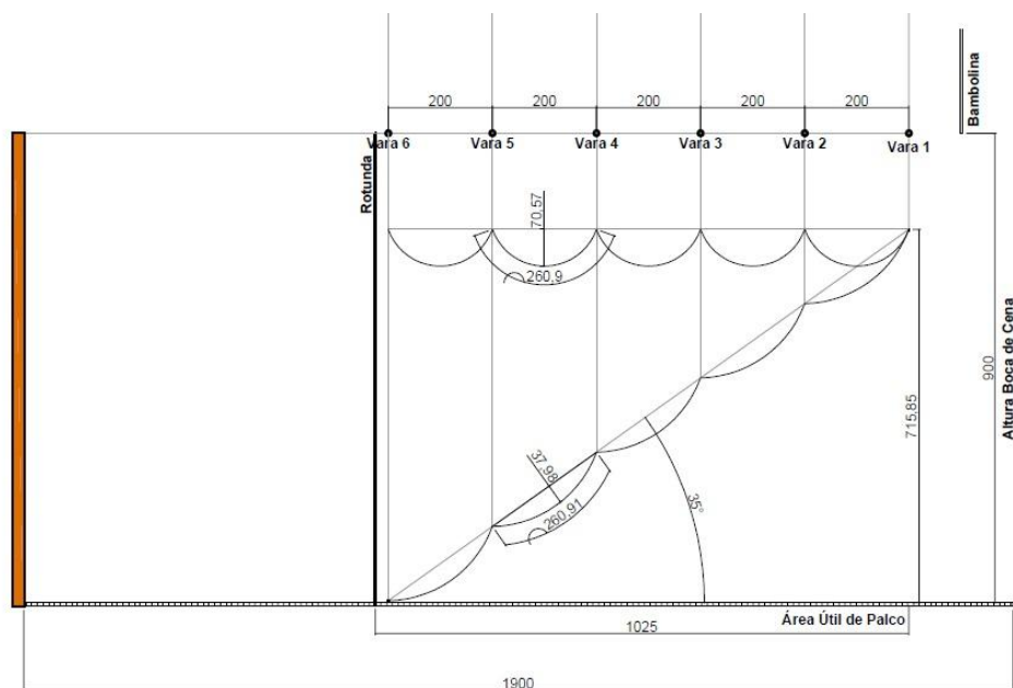
Figura 15: Segundo Corte, em software AutoCad 2007, mostrando as alturas de cada vara cônica, a inclinação de 35° na estrutura, e o abaulamento da estrutura entre cada vara cônica. Fonte: Stefanello Studio.
