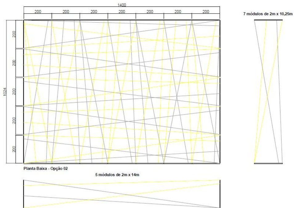
Figura 12: Segunda Proposta – planta baixa desenhada em software AutoCad 2007, com 7 faixas de 2 m x 10,25m e 5 faixas de 2 m x 14m, formando uma trama que preenche do palco de 10,24 metros de profundidade e 14 metros de largura. Fonte: Stefanello Studio .
