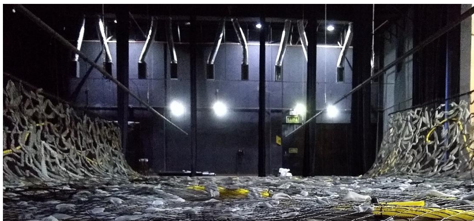
Figura 24: Estrutura cenográfica sendo fixada na primeira e na última vara cênica, por meio de fios de nylon pretos. Fonte: Stefanello Studio .
