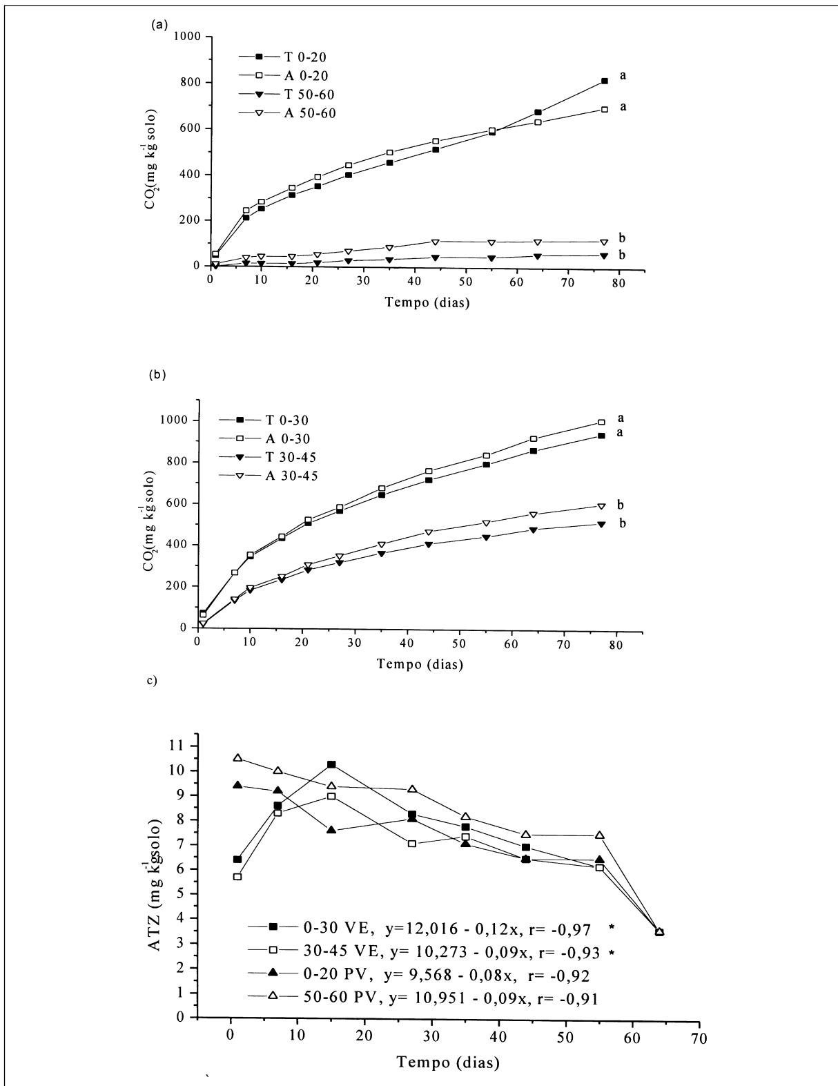
Figura 1 - Mineralização acumulada de CO 2 , ao longo do tempo, na ausência (T) e presença (A) do herbicida ATZ no solo PV (a), nas camadas 0-20 e 50-60cm, e no solo VE (b), nas camadas de 0-30 e 30-45 cm, e quantidade dessorvida de ATZ em função do tempo e em camadas dos solos PV (0-20 e 50-60cm) e VE (0-30 e 30-45cm) (c). (* Dados do 1º e 7º dia não incluídos na correlação). Médias seguidas por letras distintas diferem entre si pelo teste de Tukey a 5%.
