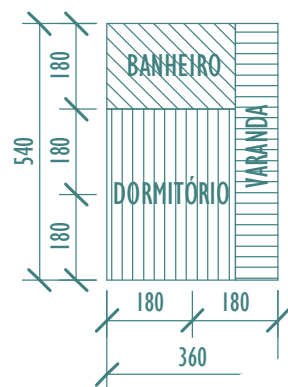
MÓDULO BASE - DORMITÓRIO
