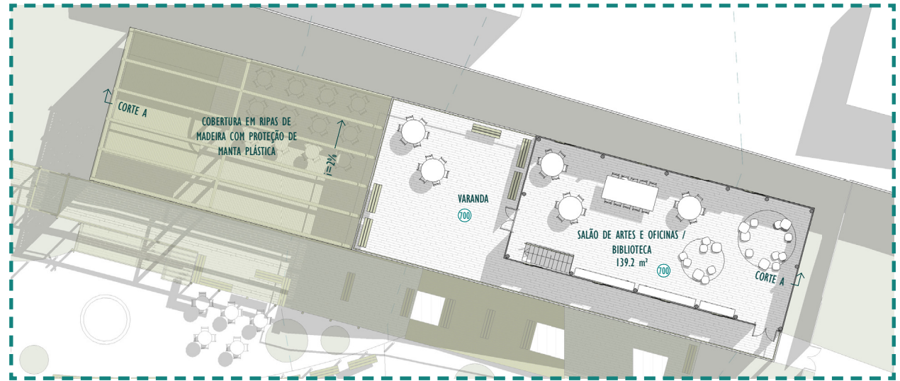
ateliê de arte segundo pavimento
