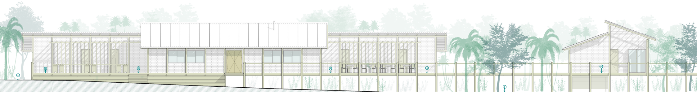
fachada frontal
