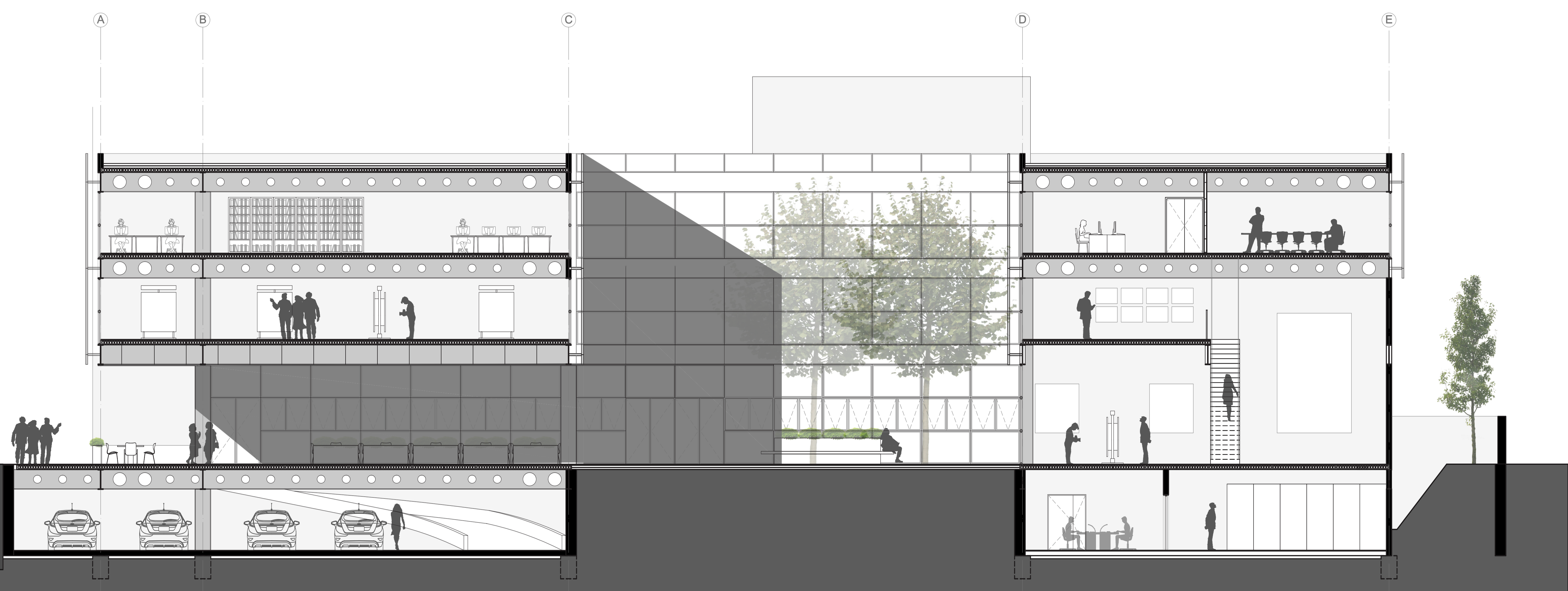
Corte AA' | 1:75
