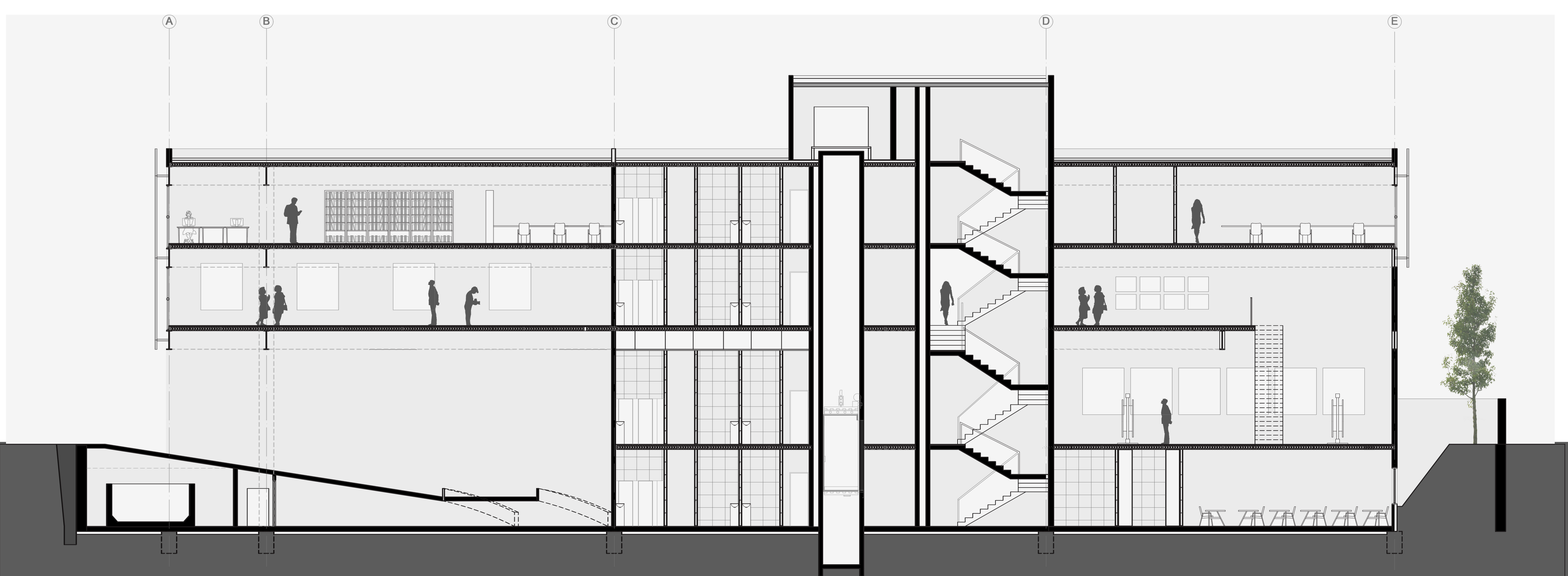
Corte BB' | 1:75
