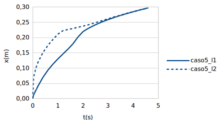
Figura 4. Curvas do escoamento da resina nas linhas I1 e I2 no caso 5.
