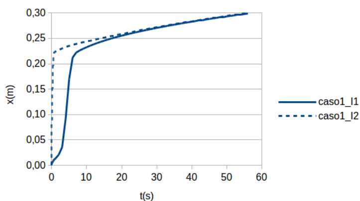
Figura 3. Posição da resina em função do tempo das linhas I1 e I2 no caso 1.
