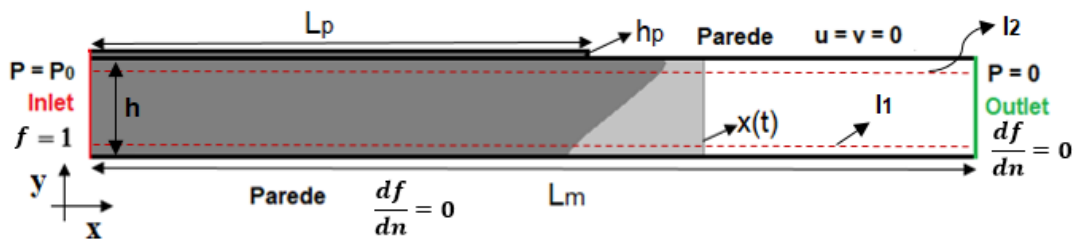
Figura 1. Domínio computacional e condições de contorno.
