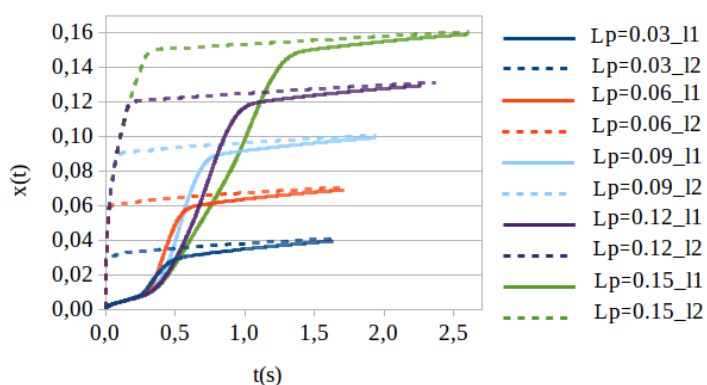
Figura 6. Curvas do escoamento da resina para os diferentes comprimentos de L_p .
