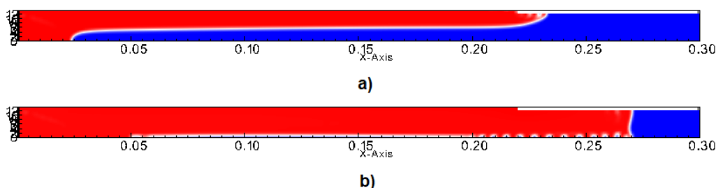
Figura 5. Escoamento da resina dentro do molde. a) no tempo de 3 s. b) no tempo de 29 s.
