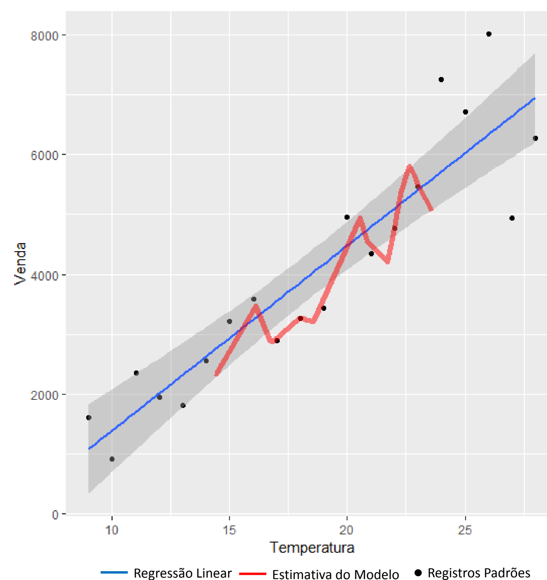
Gráfico Comparativo: Regressão Linear x Modelo Interpolação
