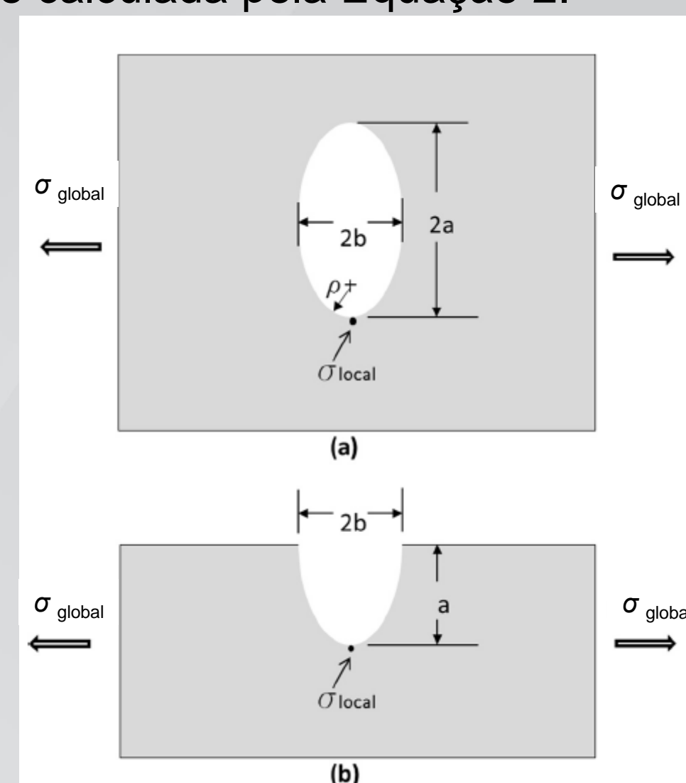
Fig. 2 – (a) Vista superior e (b) seção transversal de entalhe semi-elíptico em uma estrutura (adaptado de [6])
