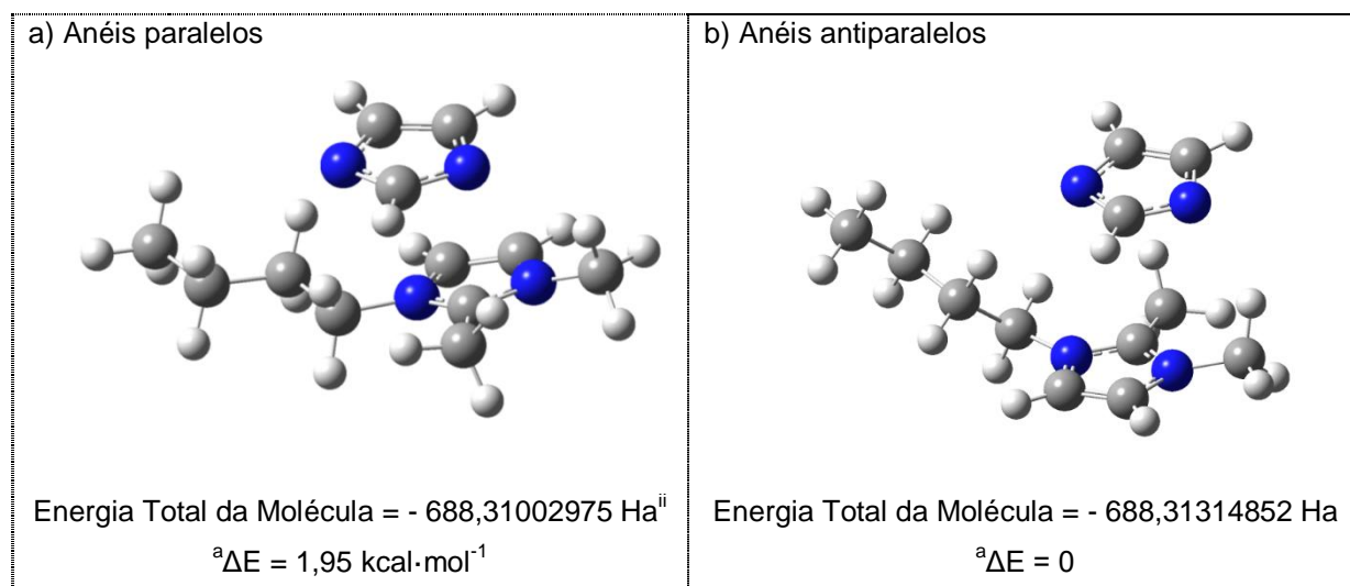
Figura 30. Estrutura otimizada obtida por cálculos de DFT ( \omega B97X-D/spaug-cc-pvtz) do par iônico BMMI-Im puro (seco): (a) com anéis imidazólicos paralelos entre si; (b) com anéis imidazólicos antiparalelos entre si. [a] Diferença energética entre as configurações, considerando a mais estável como zero.
