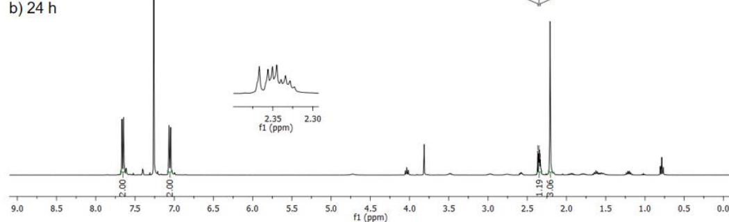
Figura A44. Espectros de RMN de ^1\text{H} (400 MHz, \text{CDCl}_3 ) da 4-metilacetofenona deuterada com \text{BMMI}\cdot\text{Pro} , 1 h (a) e 24 h(b), (Tabela 9, entrada 2b).
