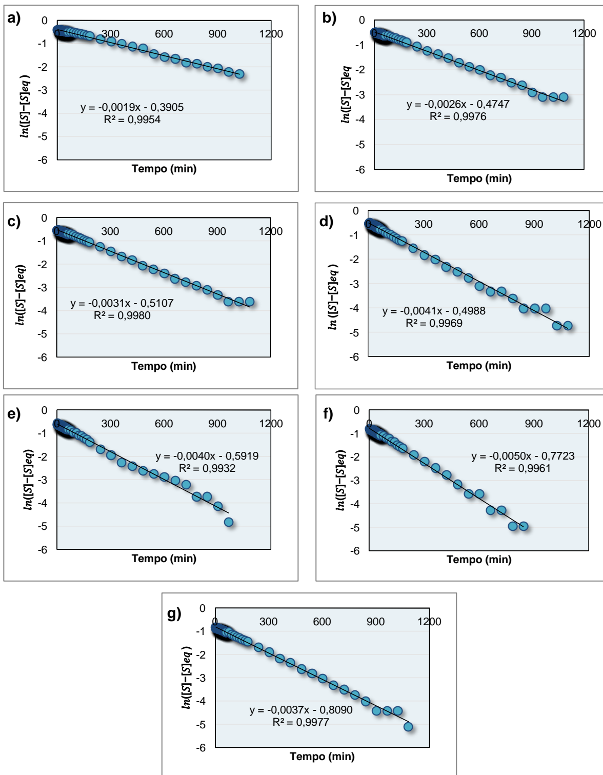
Figura 47. Equação cinética linearizada ( \ln([S] - [S]_{eq}) \times t ) das reações entre fenilacetileno e BMMI-Pro em CDCl_3 em diferentes concentrações: a) 0,9 \text{ mol}\cdot\text{L}^{-1} de substrato e 0,09 \text{ mol}\cdot\text{L}^{-1} de LI; b) 0,9 \text{ mol}\cdot\text{L}^{-1} e 0,12 \text{ mol}\cdot\text{L}^{-1} ; c) 0,9 \text{ mol}\cdot\text{L}^{-1} e 0,15 \text{ mol}\cdot\text{L}^{-1} ; d) 0,9 \text{ mol}\cdot\text{L}^{-1} e 0,18 \text{ mol}\cdot\text{L}^{-1} ; e) 0,8 \text{ mol}\cdot\text{L}^{-1} e 0,18 \text{ mol}\cdot\text{L}^{-1} ; f) 0,7 \text{ mol}\cdot\text{L}^{-1} e 0,18 \text{ mol}\cdot\text{L}^{-1} ; g) 0,6 \text{ mol}\cdot\text{L}^{-1} e 0,18 \text{ mol}\cdot\text{L}^{-1} .
