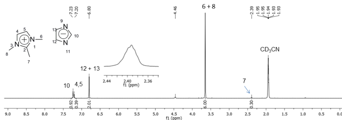
Figura A14. Espectro de RMN de ^1\text{H} (400 MHz) do MMMI·Im em \text{CD}_3\text{CN} (0,2 mol·L ^{-1} ) após 1 h.
