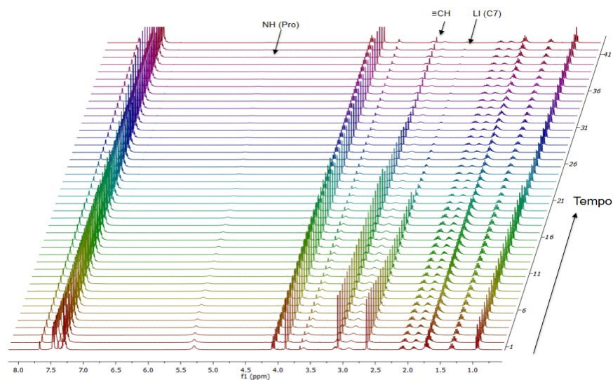
Figura 45. Resumo do monitoramento da reação entre fenilacetileno (0,9 mol·L -1 ), BMMI-Pro (0,18 mol·L -1 ) e CDCl 3 nas 8 primeiras horas de reação.
