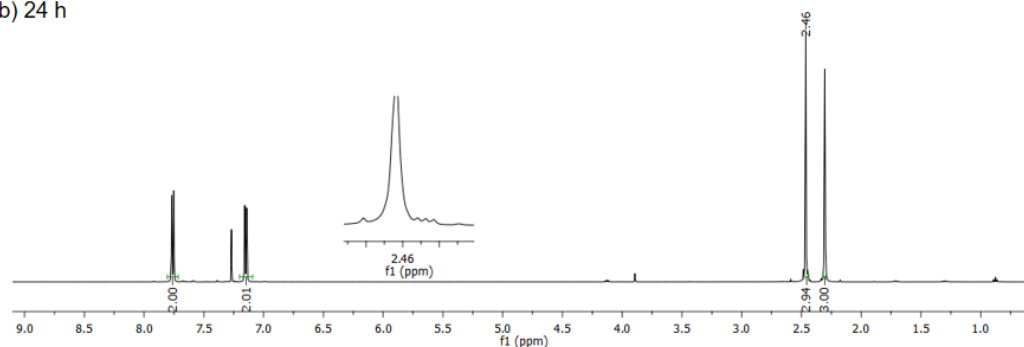
Figura A43. Espectros de RMN de ^1\text{H} (500 MHz, \text{CDCl}_3 ) da 4-metilacetofenona deuterada com \text{BMMI}\cdot\text{HCO}_3 , 1 h (a) e 24 h(b), (Tabela 9, entrada 2a).
