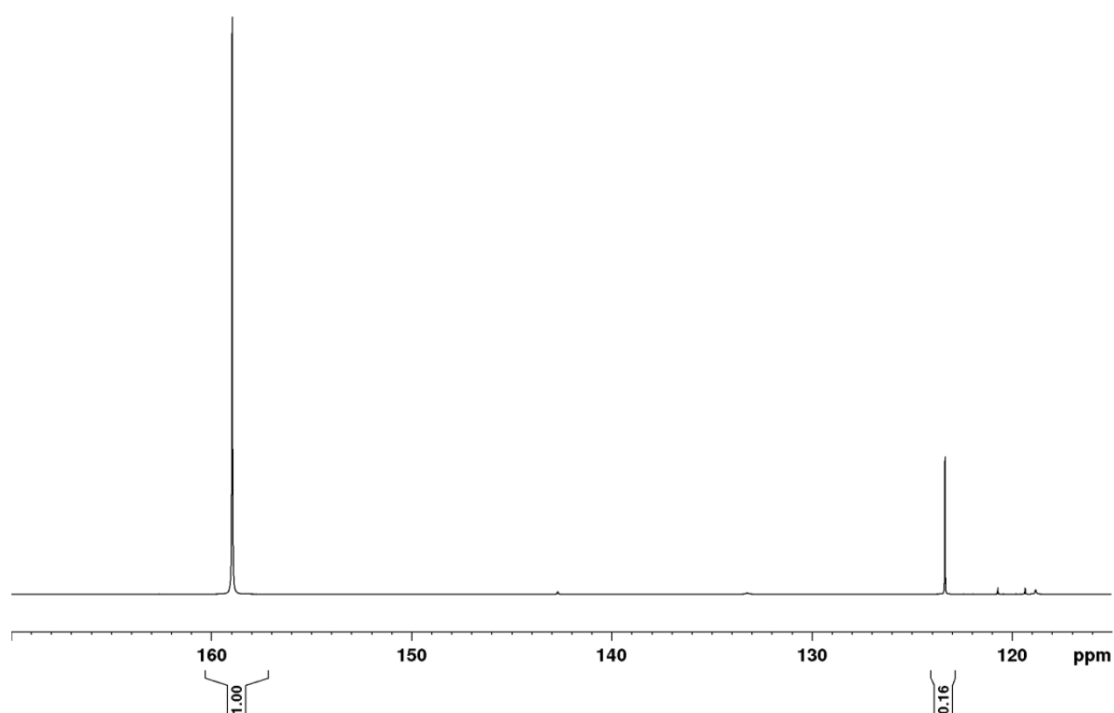
Figura A94. Espectro de RMN de ^{13}\text{C}\{-^1\text{H}\} (100 MHz) da solução de BMMI·Im/H 2 O (1/100) + ^{13}\text{CO}_2 (1 bar), (Tabela 14, entrada 6).
