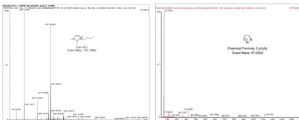
Figura A6. Espectro de ESI-HRMS BMMI-Pir em MeCN: modo positivo (esquerda), modo negativo (direita).
