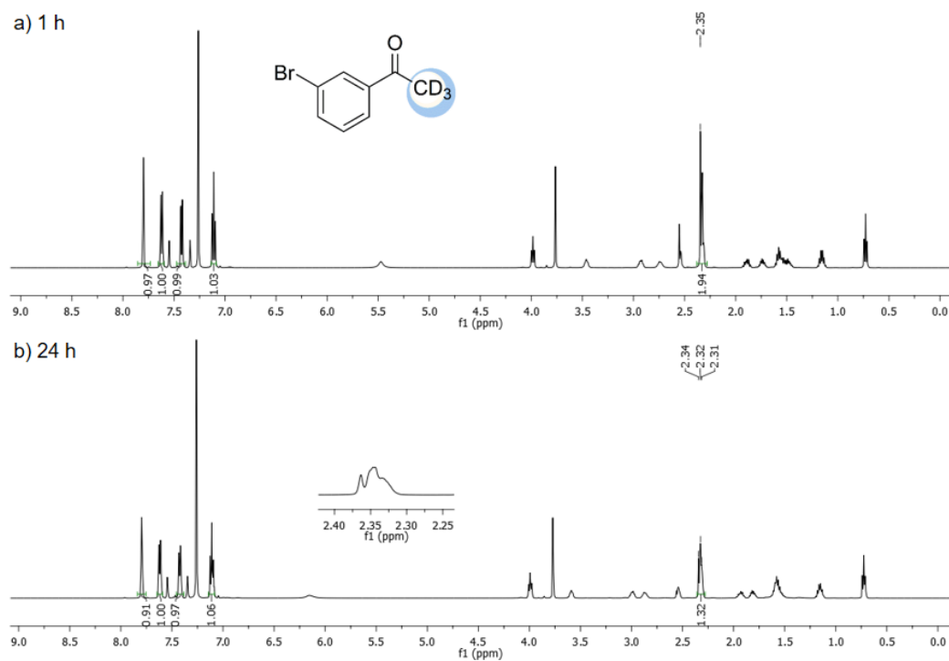
Figura A60. Espectros de RMN de ^1\text{H} (500 MHz, \text{CDCl}_3 ) da 3-bromoacetofenona deuterada com BMMI-Pro, 1 h (a) e 24 h(b), (Tabela 9, entrada 15).
