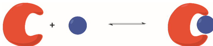
Esquema 6. Esquema gráfico para a formação do complexo hóspede (água-azul) @hospedeiro (PIC-vermelho).
