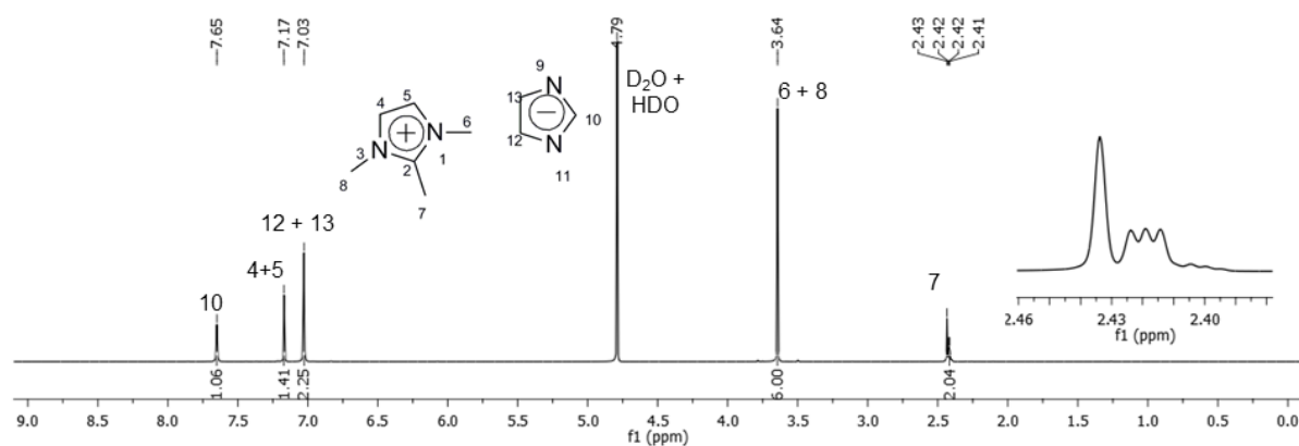
Figura A20. Espectro de RMN de ^1\text{H} (400 MHz) do MMMI-Im em \text{D}_2\text{O} (0,2 mol·L ^{-1} ) após 1 h.
