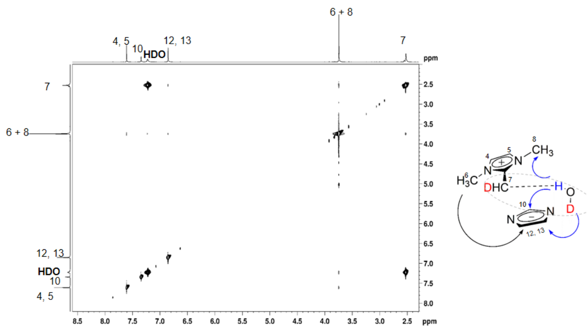
Figura A29. Mapa de contorno do espectro de ^1\text{H}, ^1\text{H} -NOESY (400 MHz) do MMMI-Im em \text{DMSO}-d_6 (1 mol·L ^{-1} ), PIC.
