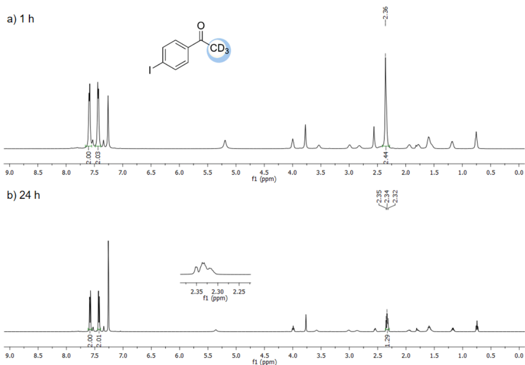
Figura A48. Espectros de RMN de ^1\text{H} (500 MHz, \text{CDCl}_3 ) da 4-iodoacetofenona deuturada com BMMI-Pro, 1 h (a) e 24 h(b), (Tabela 9, entrada 4b).
