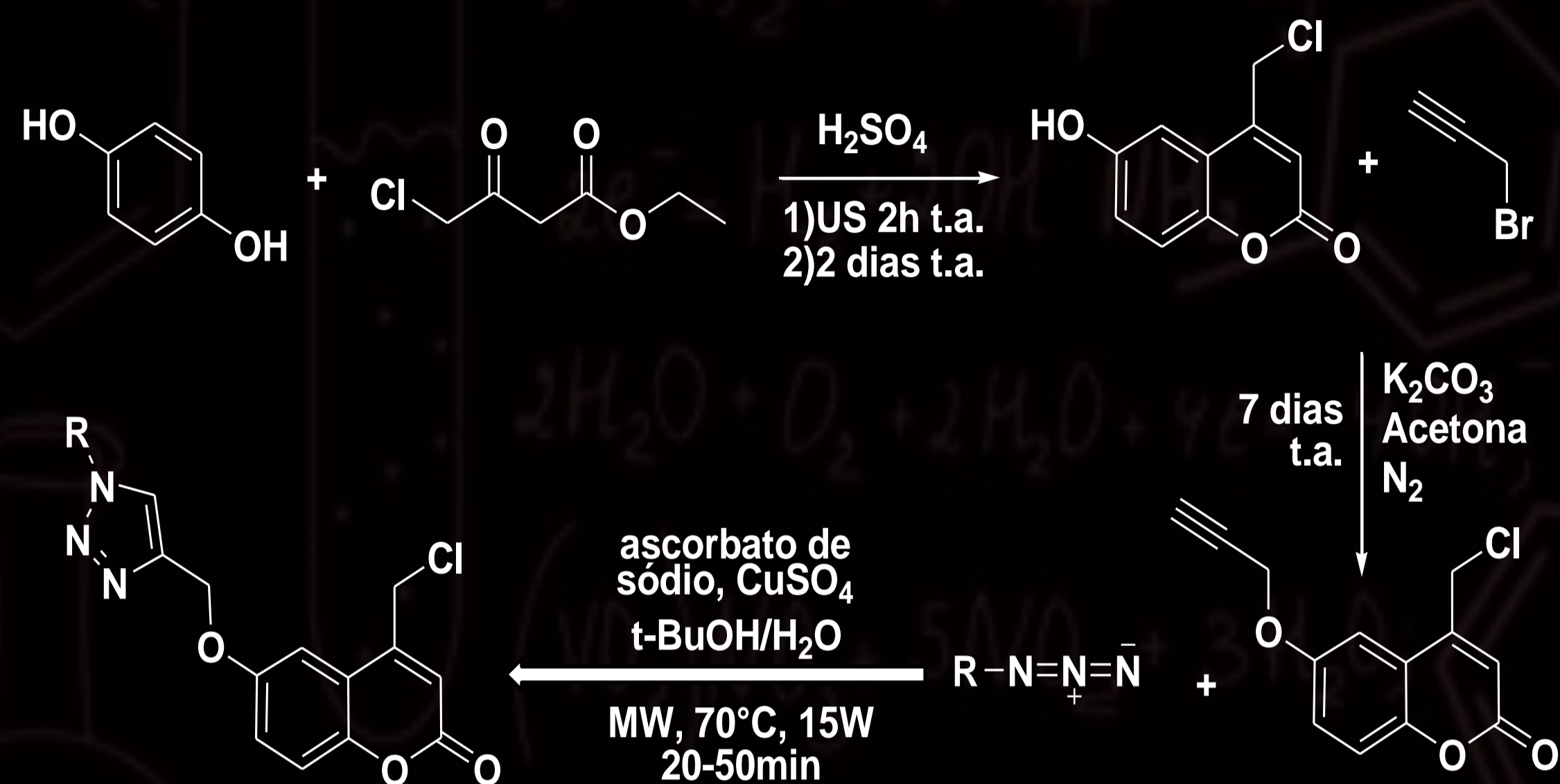
Figura 2. Rota sintética
