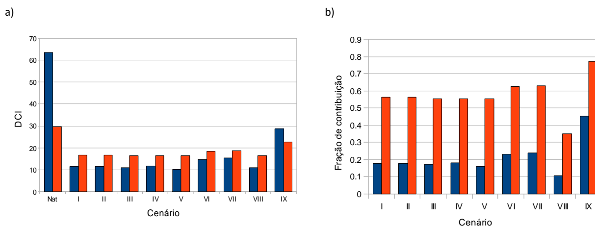
Figura 8. Simulação Fragmentos ; espécies migradoras em vermelho e residentes em azul: a) comparação dos valores de DCI entre os cenários; b) contribuição das barreiras naturais para o DCI total da bacia.
