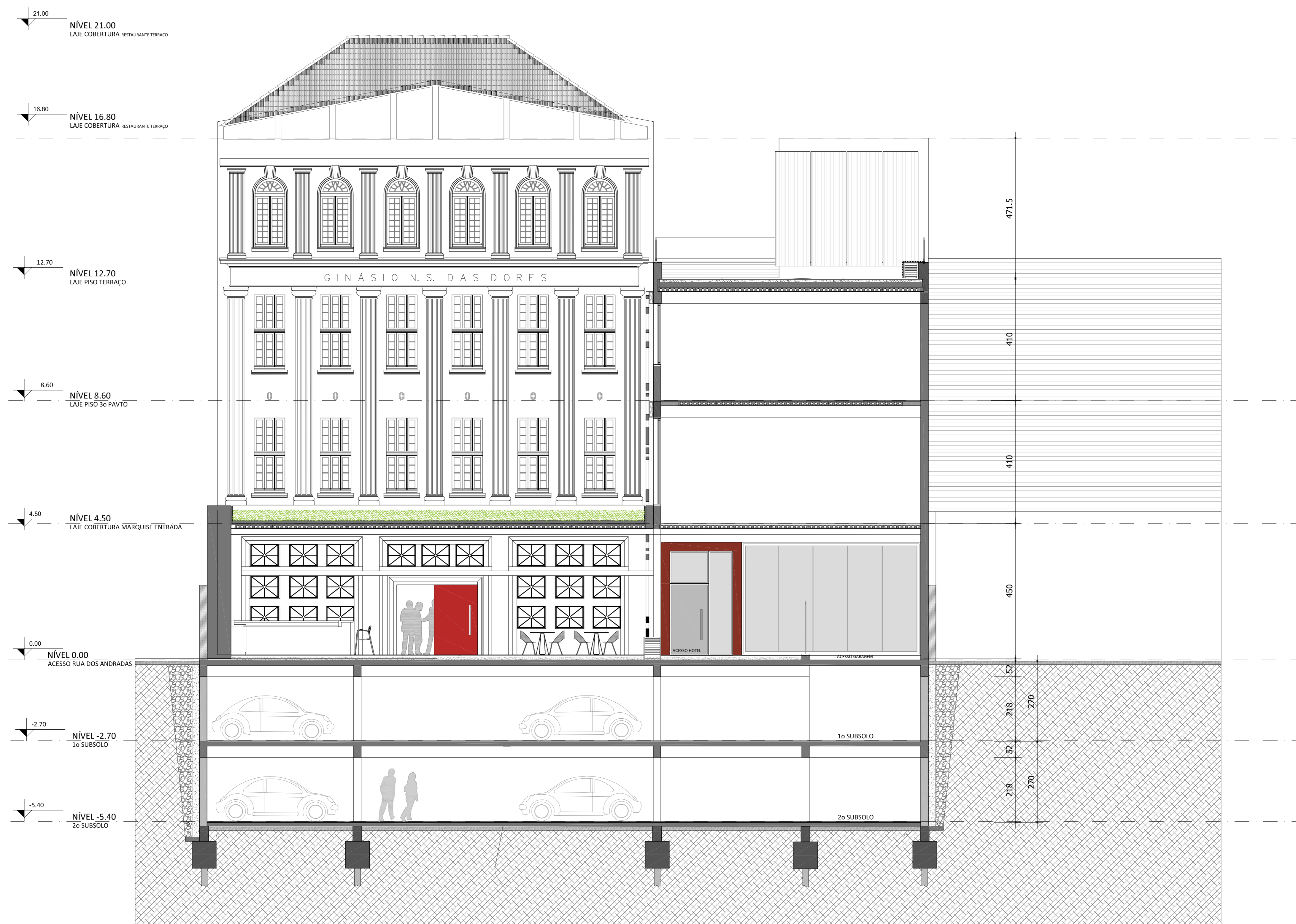
CORTE AA_esc 1/75
