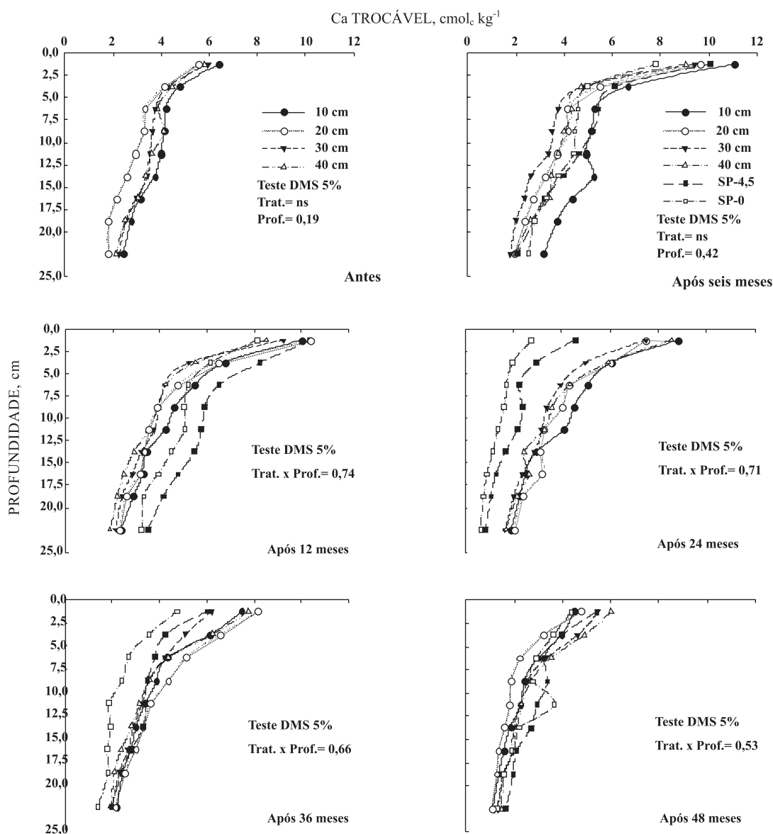
Figura 2. Teor de cálcio trocável em diferentes épocas da aplicação superficial de calcário em Latossolo Vermelho, sob sistema plantio direto e integração lavoura-pecuária, com diferentes pressões de pastejo no inverno (ns: não significativo).
