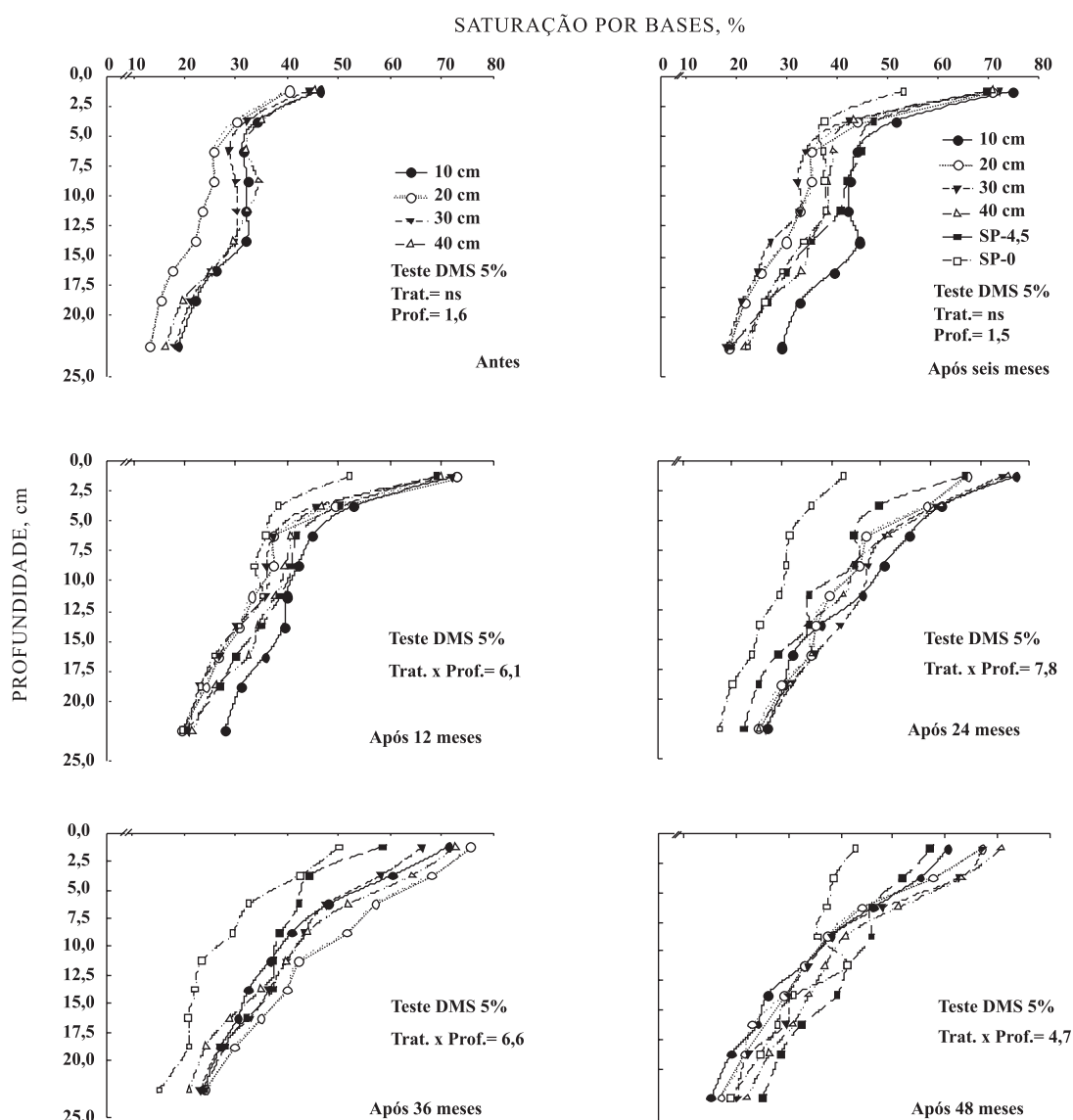
Figura 4. Valores de saturação por bases em diferentes épocas da aplicação superficial de calcário em Latossolo Vermelho, sob sistema plantio direto e integração lavoura-pecuária, com diferentes pressões de pastejo no inverno (ns: não significativo).
