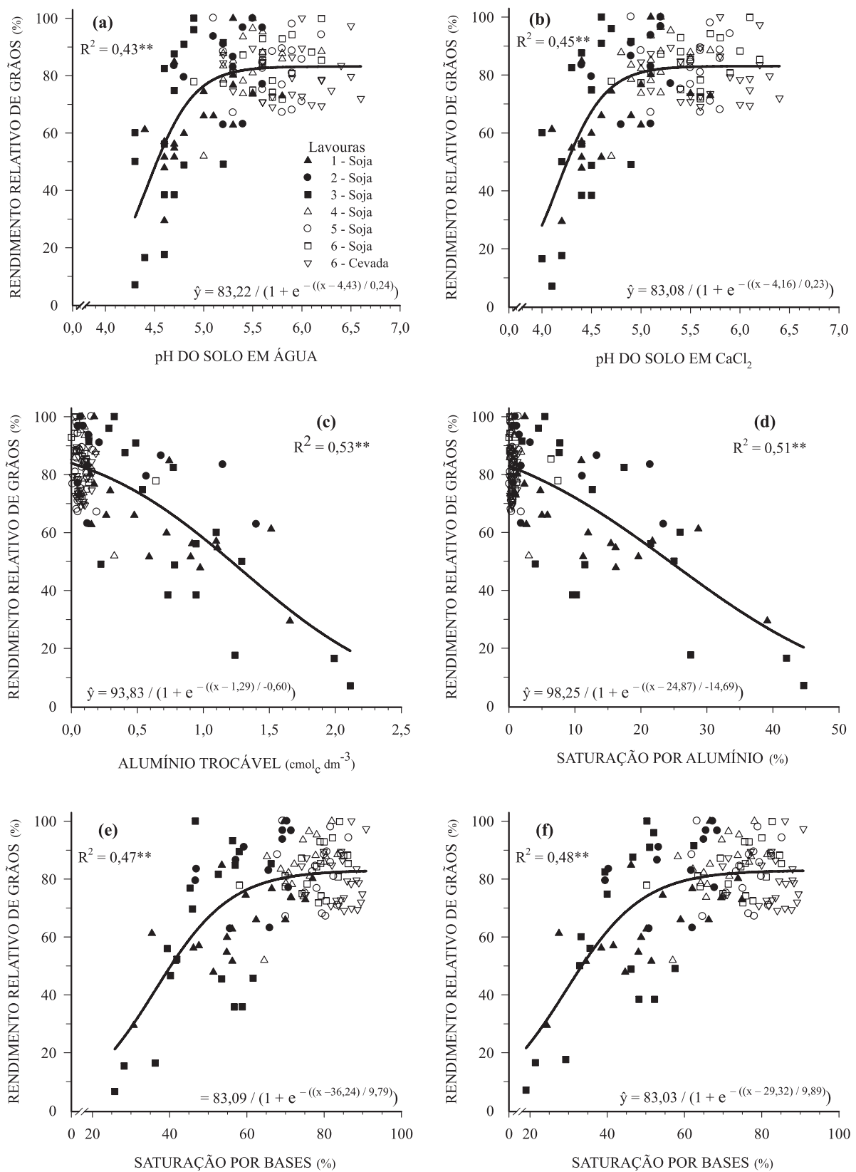
Figura 2. Relação entre o rendimento relativo de grãos e os indicadores de acidez do solo na camada de 0 a 10 cm de profundidade em lavouras no sistema plantio direto: (a) pH em água; (b) pH em CaCl 2 ; (c) alumínio trocável; (d) saturação por alumínio e saturação por bases; (e) Eq. Escosteguy & Bissani (1999) e (f) Eq. Kaminski et al. (2001).
