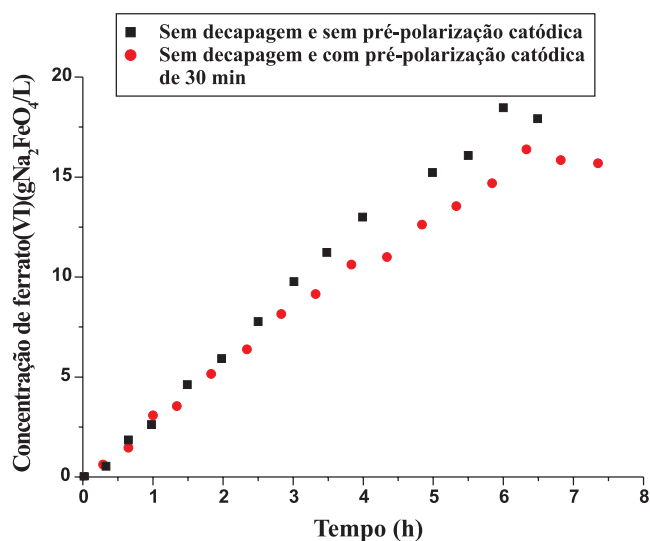
Figura 4. Influência da pré-polarização catódica do ânodo na concentração de ferrato(VI) (ânodo de ferro gusa em NaOH 10 mol/L). Comparação dos tratamentos: a) sem decapagem e sem pré-polarização catódica e b) sem decapagem e com pré-polarização catódica de 30 min
