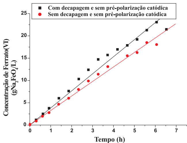
Figura 5. Influência da decapagem do ânodo na concentração de ferrato(VI) (ânodo de ferro gusa em NaOH 10 mol/L). Comparação dos tratamentos: a) sem decapagem e sem pré-polarização catódica e b) com decapagem e sem pré-polarização catódica
