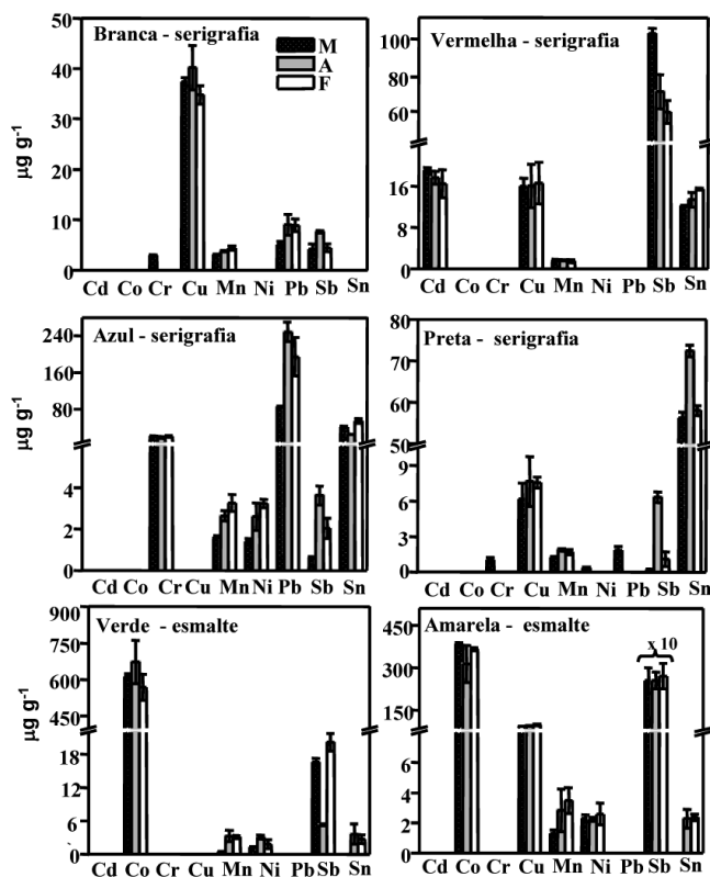
Figura 1. Concentrações dos elementos determinadas por ICP-MS nas tintas. M: decomposição em copo de quartzo com aquecimento em forno de microondas; A: decomposição com \text{HNO}_3 e calcinação em copo aberto e F: decomposição com \text{HF} + \text{HNO}_3 e calcinação em cadinho de Pt. Os resultados são expressos em \mu\text{g g}^{-1} e as barras de erro representam o desvio padrão de três determinações. A ausência de barras indica que os elementos não foram detectados na amostra
