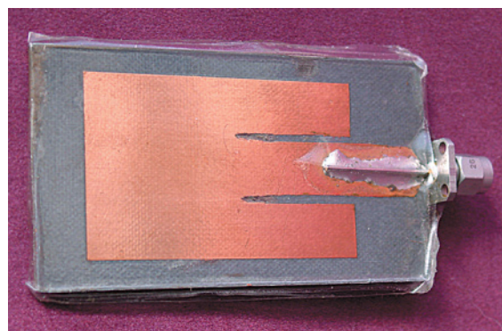
Figura 7. Antena tipo patch retangular medida. Figure 7. Measured Patch antenna.
