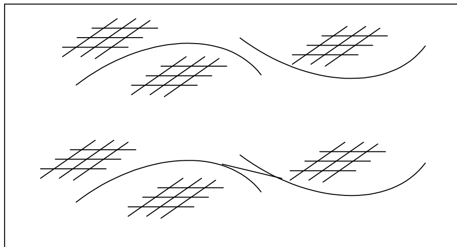
Figura 8. Curvas de raio longo concordadas com tangentes curtas
