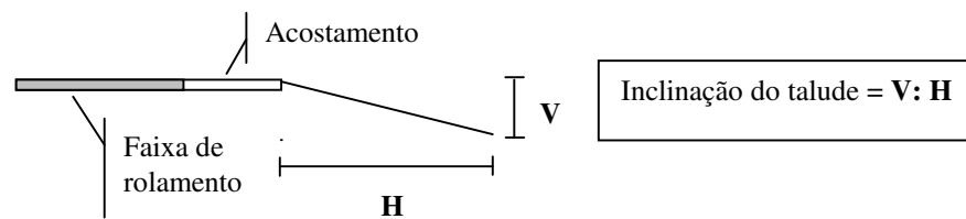
Figura 12. Perfil da área marginal da rodovia
