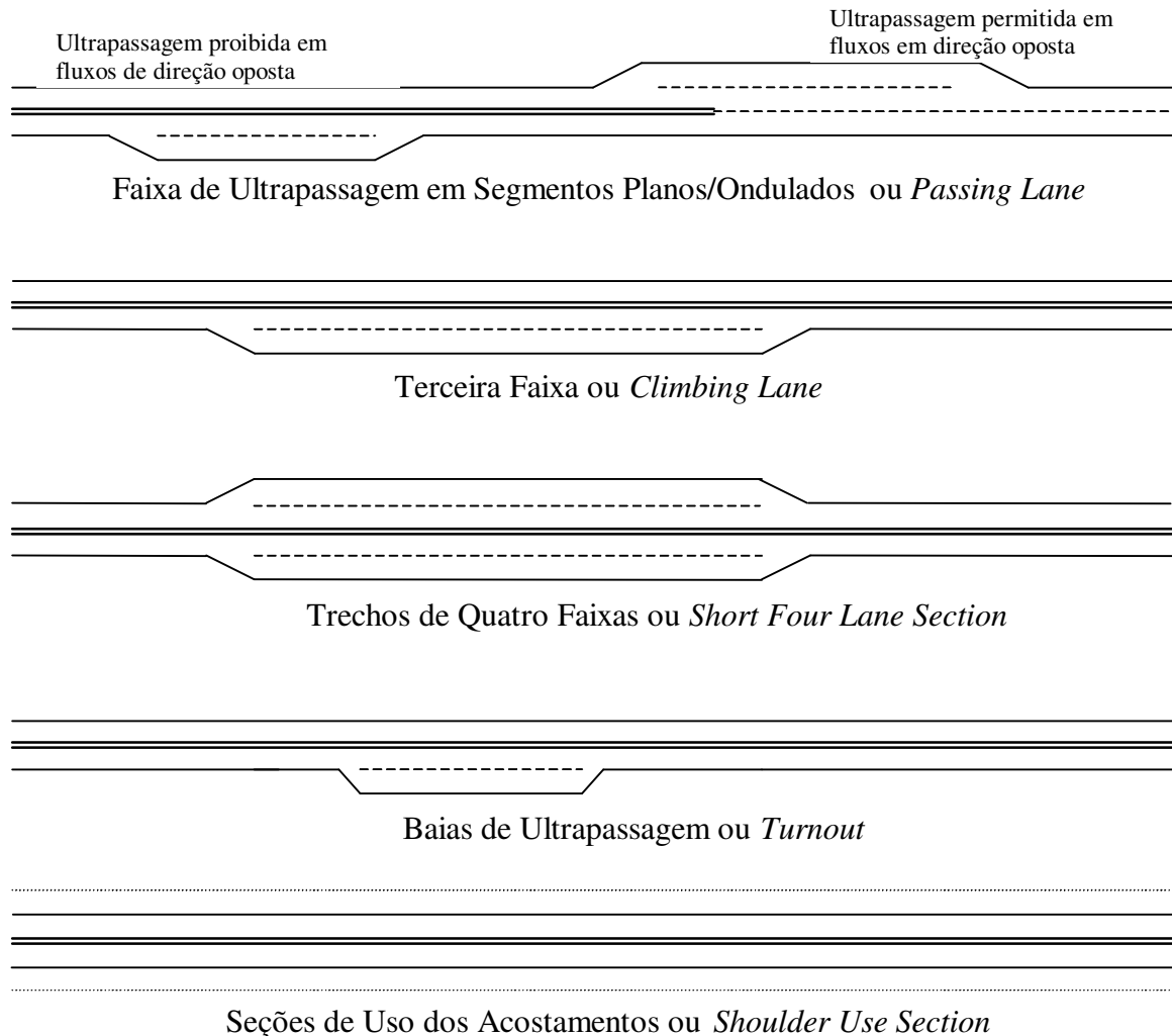
Figura 11. Tratamentos para aumentar oportunidades de ultrapassagem em rodovias rurais de pista simples
