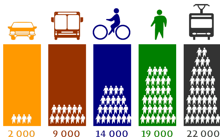
Figura 6: pessoas por hora em uma via com 3,5 m de largura (adaptado de BOTMA; PAPENDRECHT 2 , 1991 apud INTERFACE FOR CYCLING EXPERTISE, 2009, p. 7)
