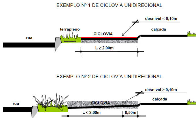
Figura 27: larguras mínimas de ciclovias unidirecionais (BRASIL, 2001b, p. 41)
