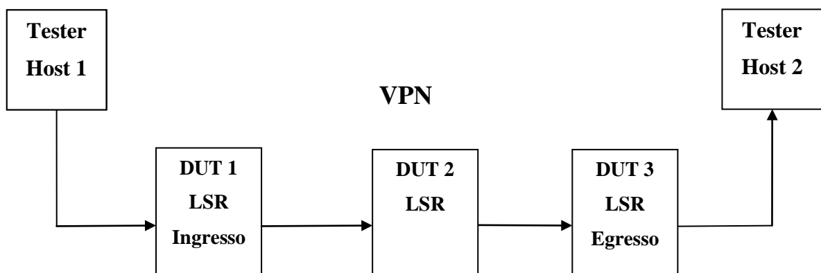
Figura 16 - Topologia para benchmark
