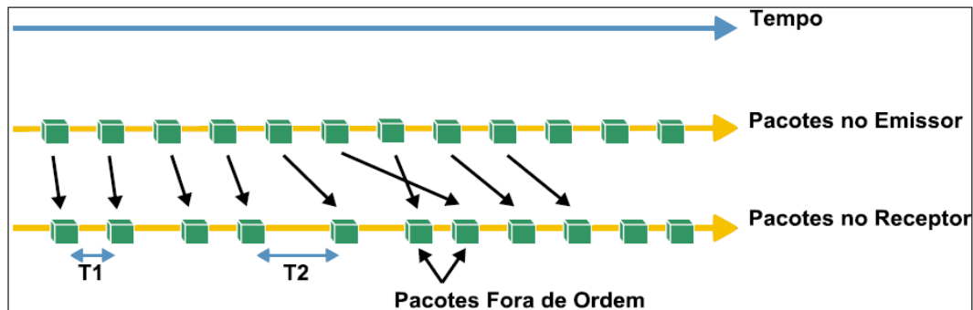
Figura 13 - Efeito do Jitter para aplicações
