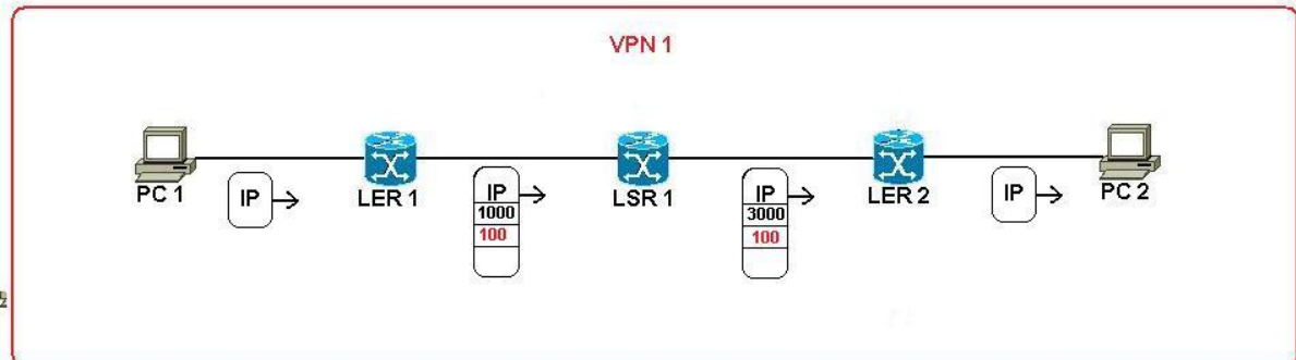
Figura 15 - Topologia para experimento
