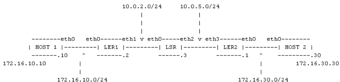
Figura 29 -Topologia após configuração
