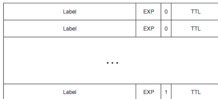
Figura 6 - Pilha de Labels
