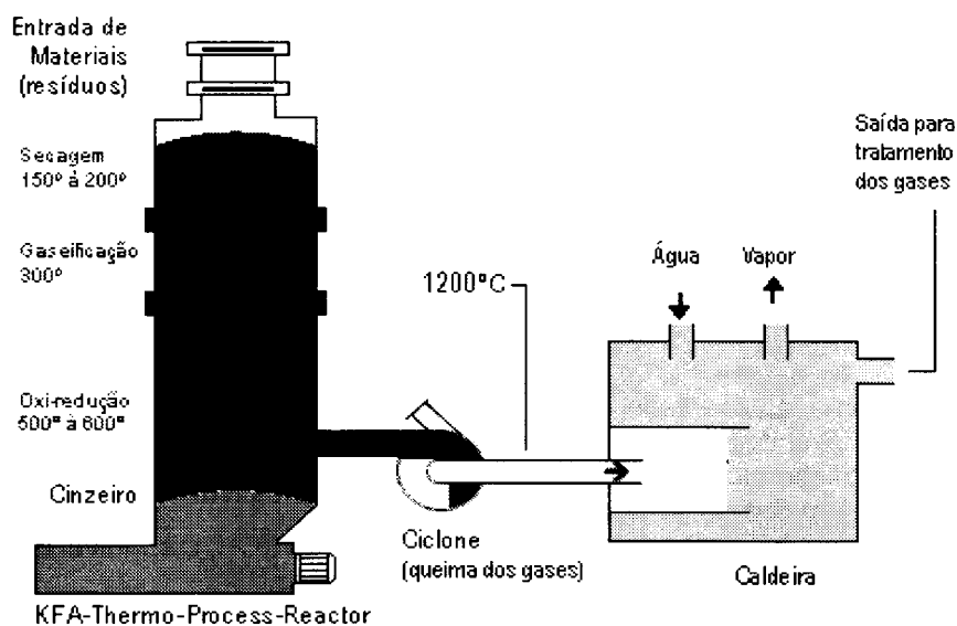
Figura 1. Desenho esquemático de um incinerador
