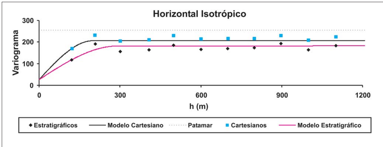
Figura 2 - Variograma horizontal isotrópico e seu modelo.
