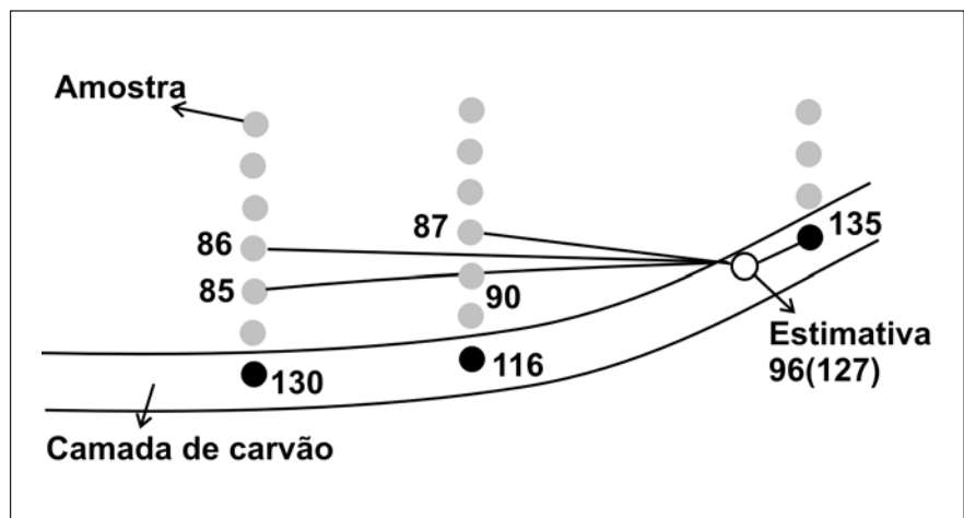
Figura 4 - Esquema de como foram realizadas algumas estimativas em coordenadas cartesianas e comparação entre os valores de uma estimativa obtida por coordenadas cartesianas (96) e de uma estimativa obtida por coordenadas estratigráficas (127).
