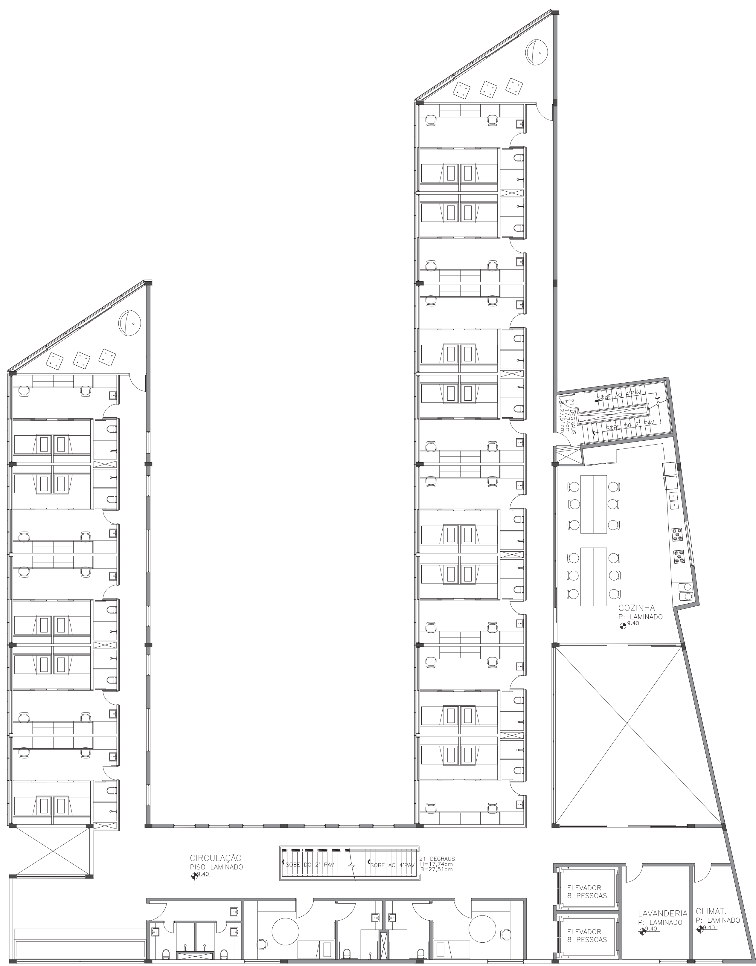
PLANTA 3° AO 8° e 10° PAVIMENTO ESCALA 1/125
