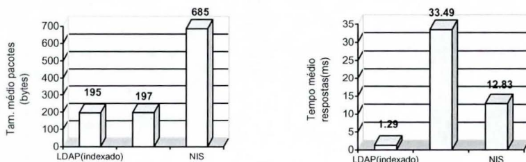
Figura 2 – LDAP versus NIS: tamanho médio dos pacotes
