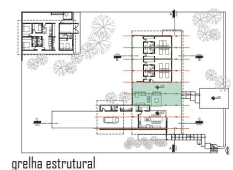
grelha estrutural
