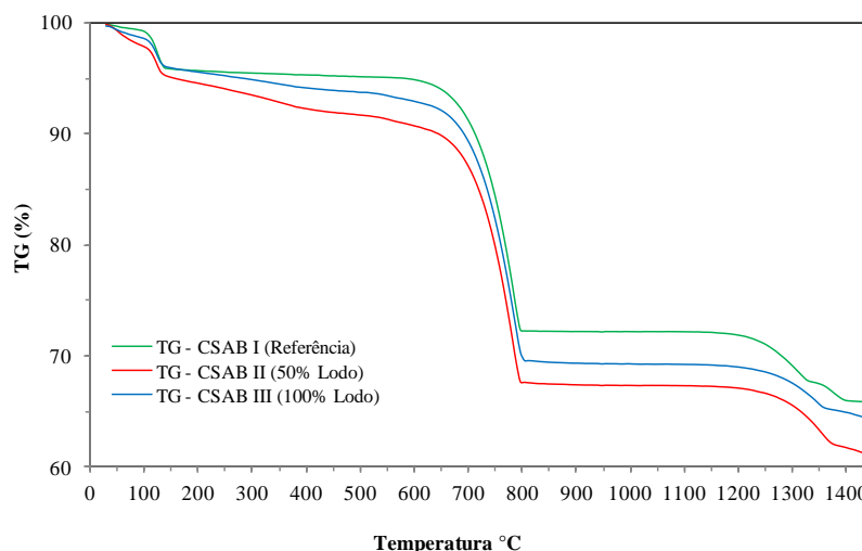
Figura 2: Curva TG das farinhas sob atmosfera de nitrogênio e taxa de aquecimento de 10°C/min.
