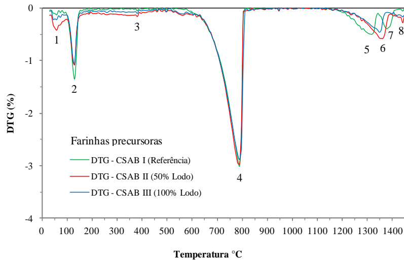
Figura 3: Curvas DTG das farinhas sob atmosfera de nitrogênio e taxa de aquecimento de 10°C/min.
