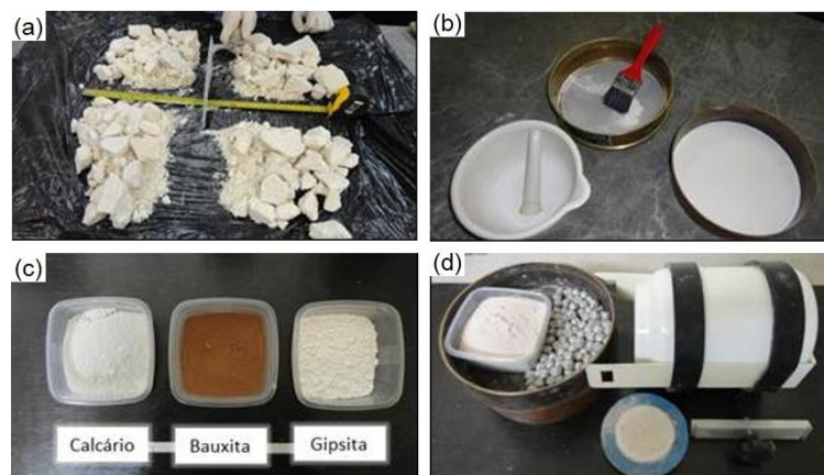
Figura 1: Quarteamento do LAA (a). Amostra do LAA seco, peneirado e usado para substituir a bauxita (b), matérias primas convencionais (c), e Farinha após o processo de mistura das matérias primas (d).
