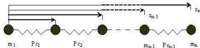
Figure 10 Riera Method. (Riera, 1980)
