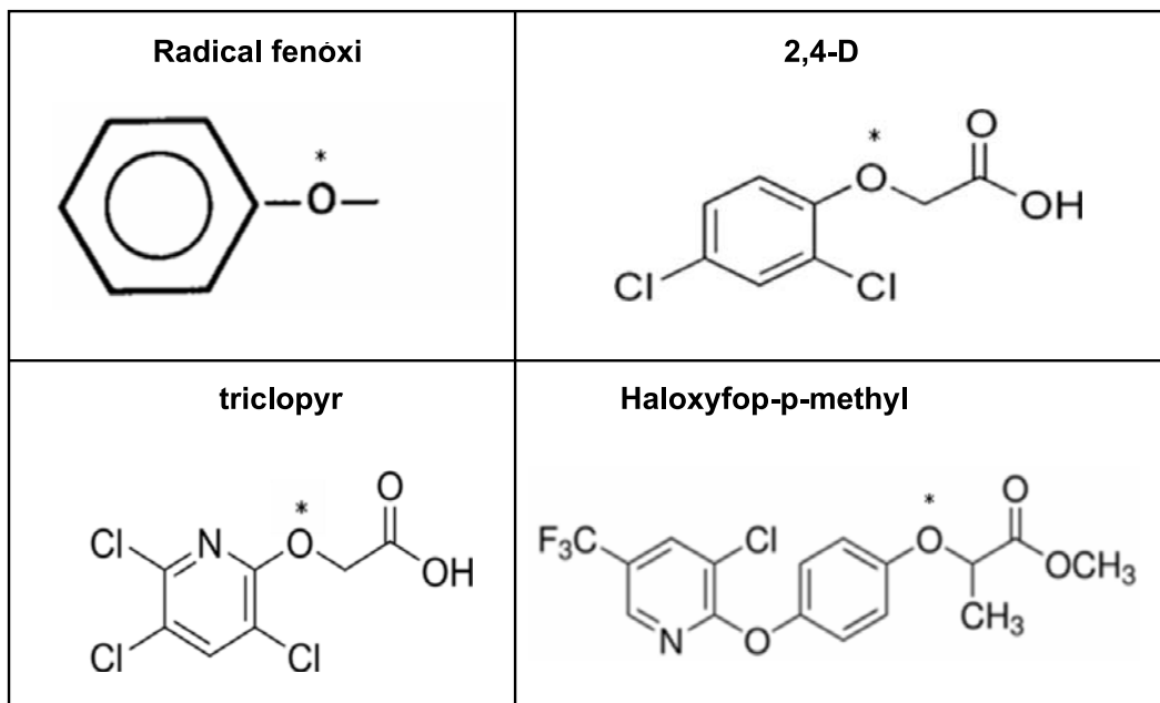
Figura 1 - Estrutura química dos herbicidas auxínicos 2,4-D e triclopyr em comparação com o herbicida inibidor da ACCase haloxypop-p-methyl. O asterisco denota a região de hidroxilação das moléculas pela ação das enzimas ariloxiacanoato dioxigenases (AADs).
