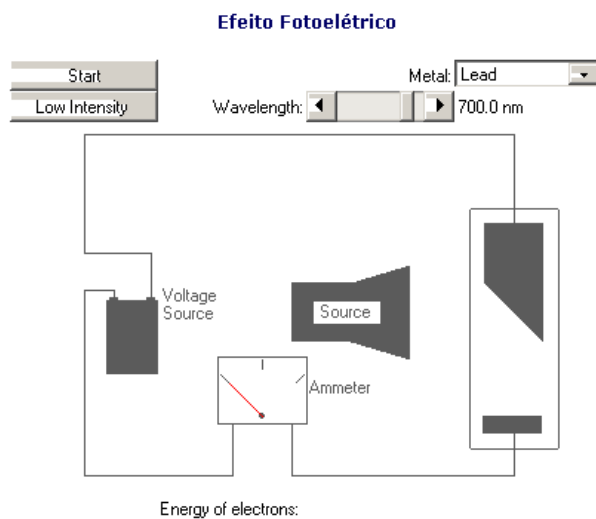
Figura 6 - Tela inicial do simulador do efeito fotoelétrico disponibilizado no material.
