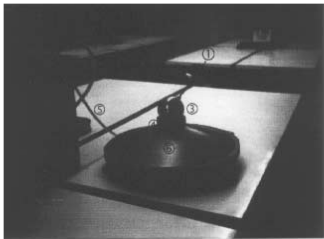
Figura 1. Uma visão esquemática do giroscópio utilizado. (1) Haste de alumínio (removível); (2) peso que encaixa na haste; (3) esfera de aço; (4) superfície de contato com a esfera, sem atrito devido à saída de ar comprimido; (5) entrada de ar comprimido; (6) base de sustentação.
